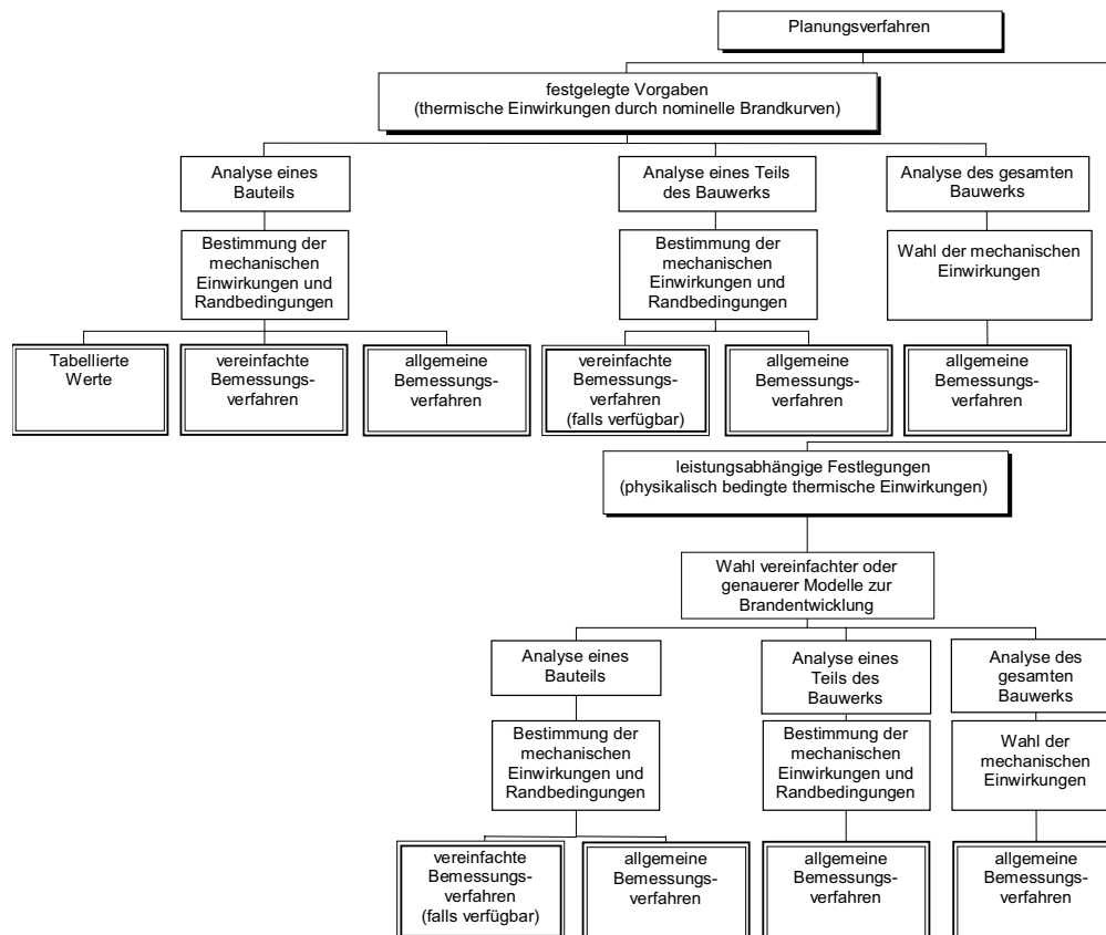
Bild 1 — Alternative Bemessungsverfahren
