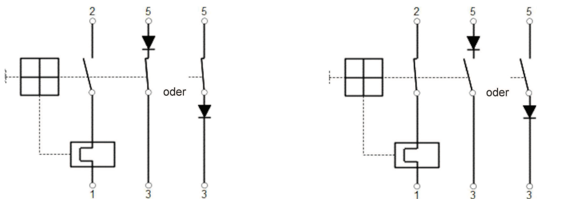
a) Druckknopf freigegeben: Schutzschalter ist offen, Signalkontakt ist geschlossen
