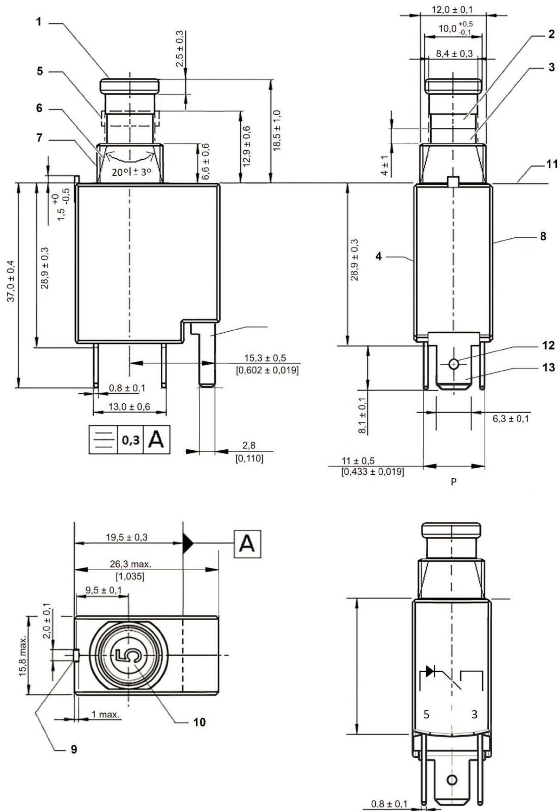
a) Standard-Druckknopf (S)
