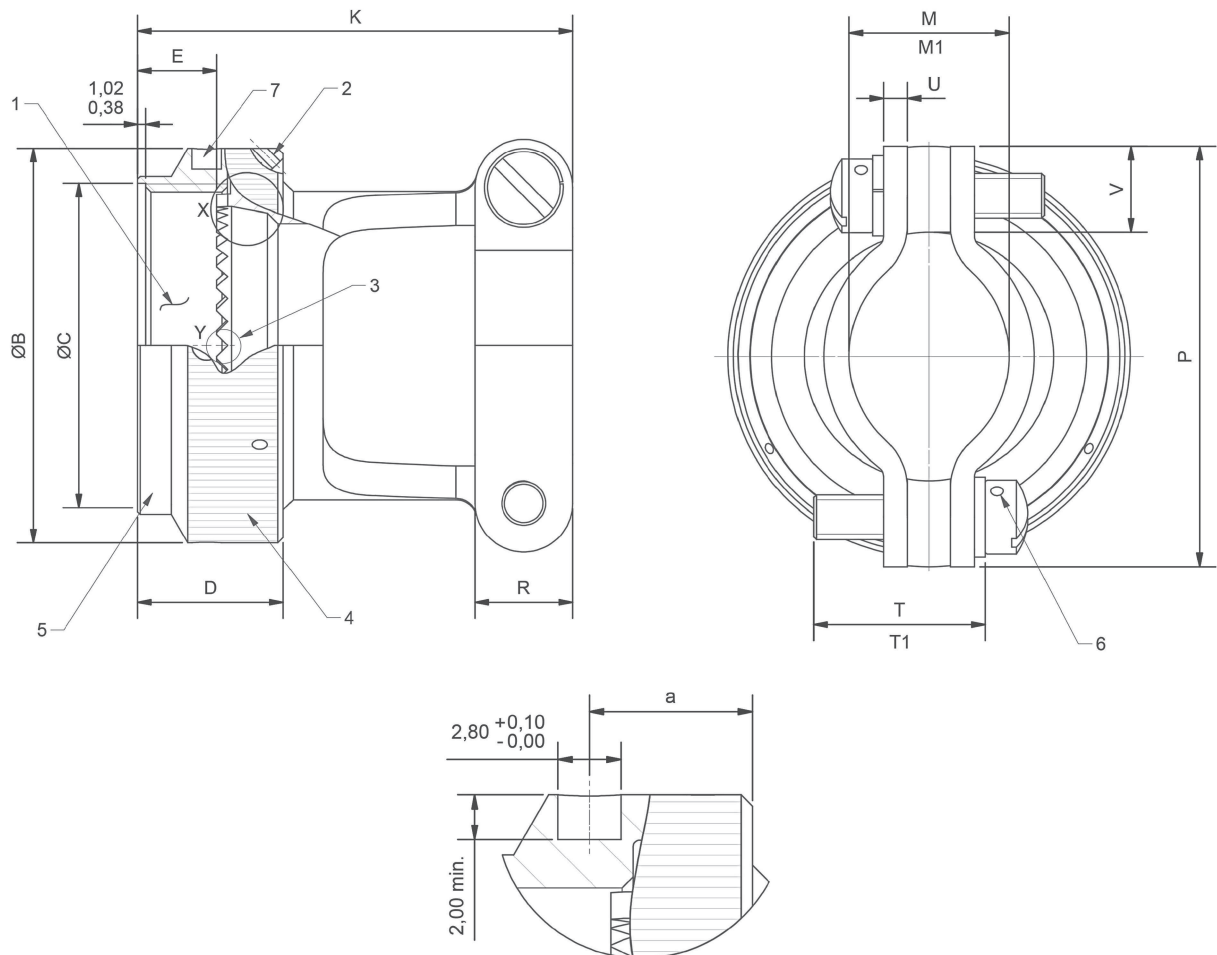
Einzelheit Z
