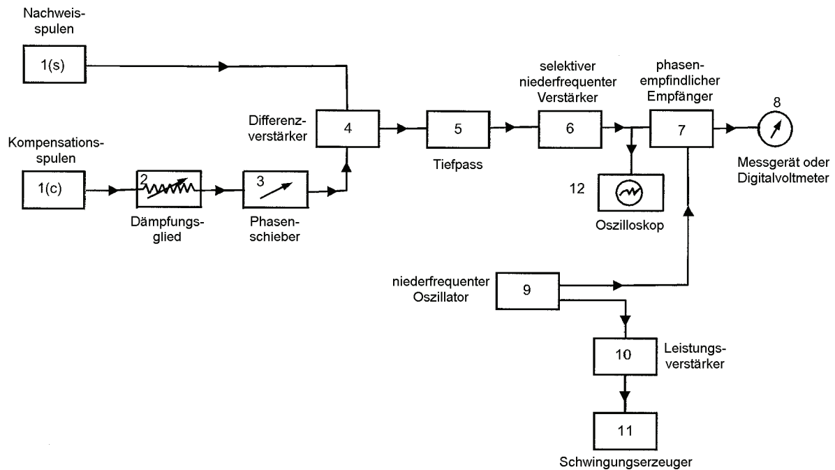
Bild 3 – Messeinrichtung (VCM)
