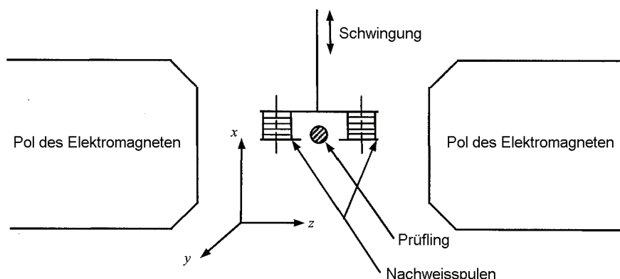
Bild 1 – Schwingsspulenmethode – Anordnung von Prüfling und Spulen
