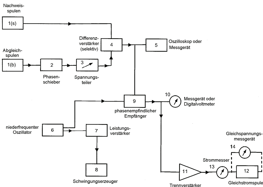
Bild 5 – Messeinrichtung (VSM)
