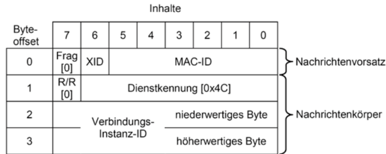
Bild 10 – Format der Anforderung, eine Verbindung zu schließen
