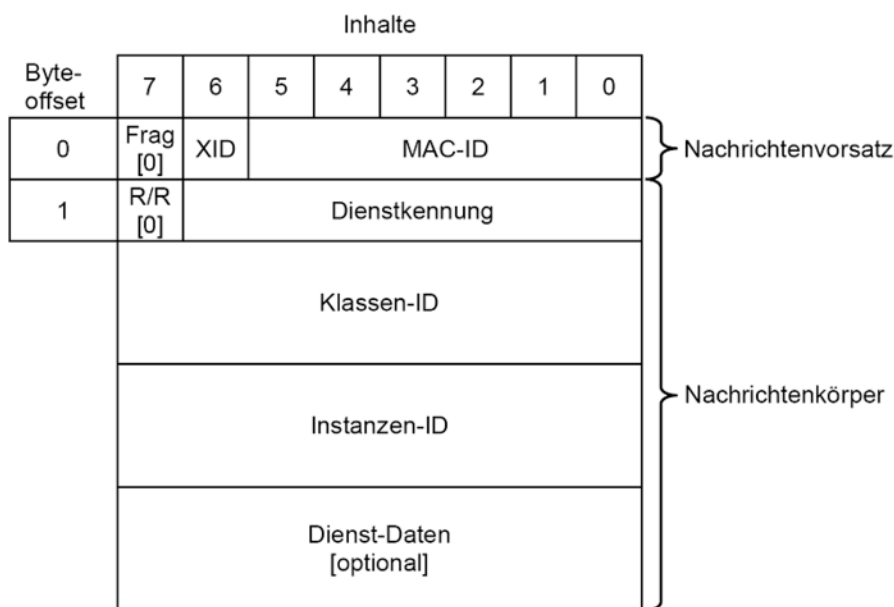
Bild 12 – Format der nicht fragmentierten expliziten Anforderungsnachricht, Werte 0–3
