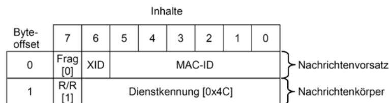
Bild 11 – Format der Antwort, eine Verbindung zu schließen
