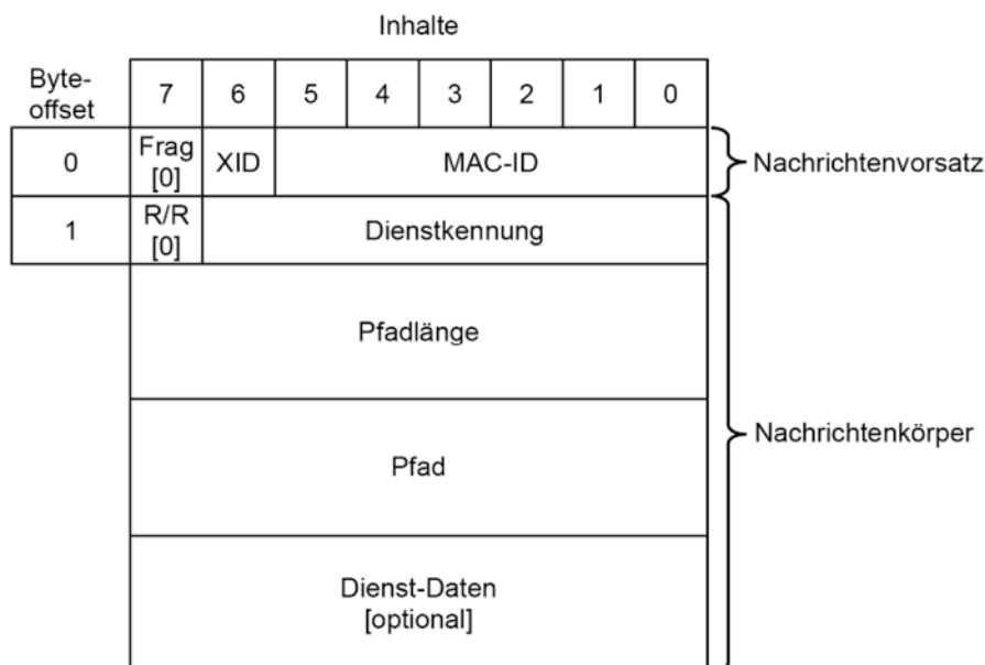
Bild 13 – Format der nicht fragmentierten expliziten Anforderungsnachricht, Wert 4
