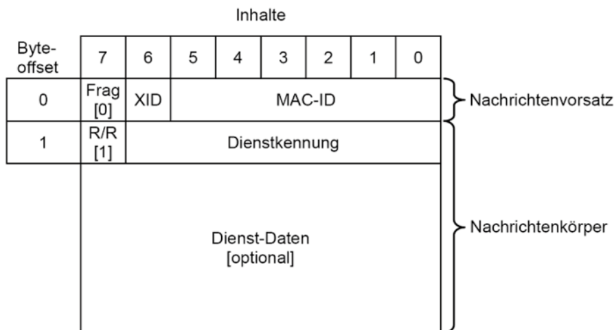
Bild 14 – Format der nicht fragmentierten erfolgreichen Antwortnachricht
