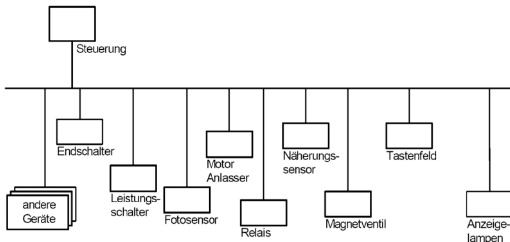
Bild 1 – Typisches DeviceNet-Steuerung-Geräte-Netzwerk
