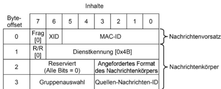
Bild 8 – Format der Anforderungsnachricht zum Öffnen einer expliziten Nachrichtenverbindung
