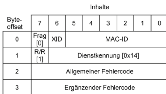
Bild 15 – Fehlerantwortnachricht
