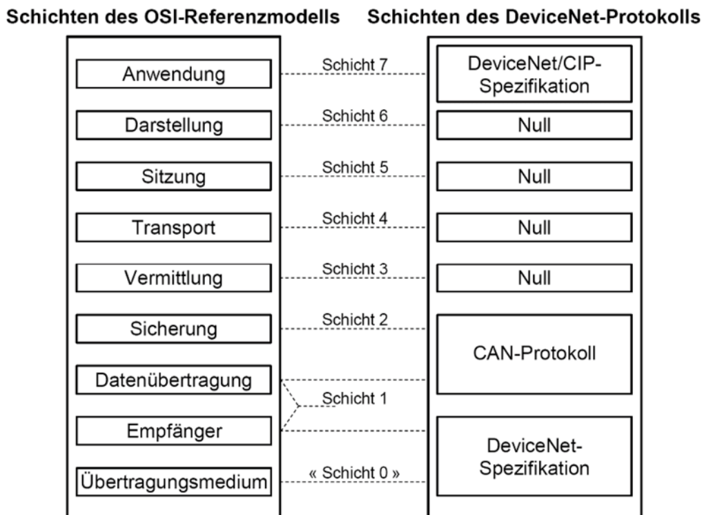
Bild 2 – Architektur des DeviceNet-Protokolls im Vergleich zum OSI-Referenzmodell
