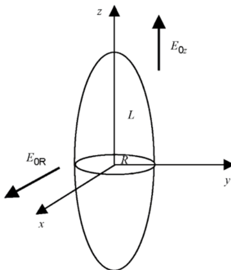
Bild 7 – Dem elektrischen Feld ausgesetztes leitendes Sphäroid
