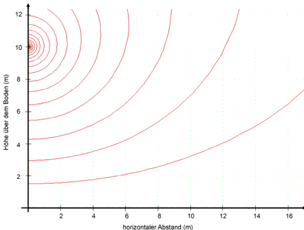
Bild 2 – Potentiallinien des elektrischen Felds, das durch einen unter Spannung stehenden Leiter bei Abwesenheit irgendwelcher Gegenstände erzeugt wird
