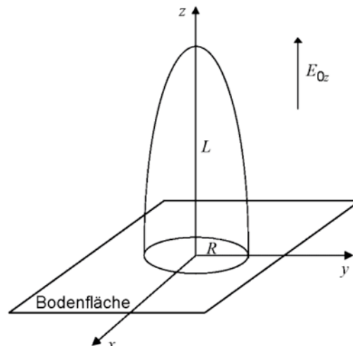
Bild 4 – Schema des halben Sphäroids, das einen auf einer Fläche, deren Potential gleich null ist, stehenden menschlichen Körper nachbildet
