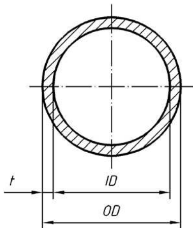
Bild 1 — Rundrohr
