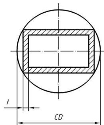
Bild 2 — Umschlingungskreis für Rohre, ausgenommen Rundrohre
