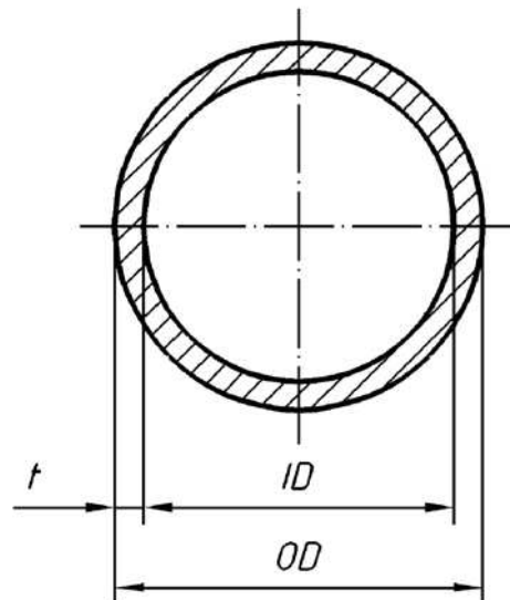
Bild 1 — Rundrohr
