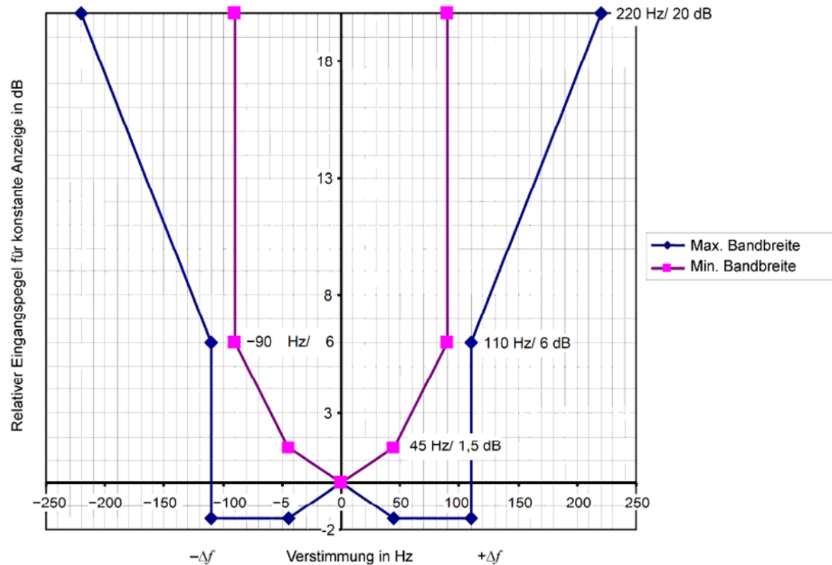
Bild 1 – Grenzen der Gesamt-Selektionskurve – Durchlassbereich (Band A)
