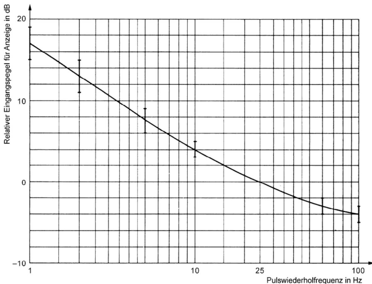
Bild 6 – Pulsbewertungskurve (Band A)
