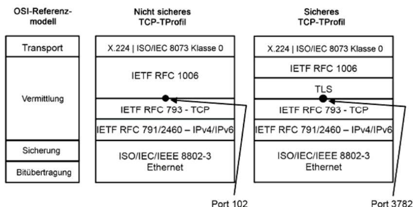
Bild 2 – T-Profile mit und ohne TLS-Schutz
