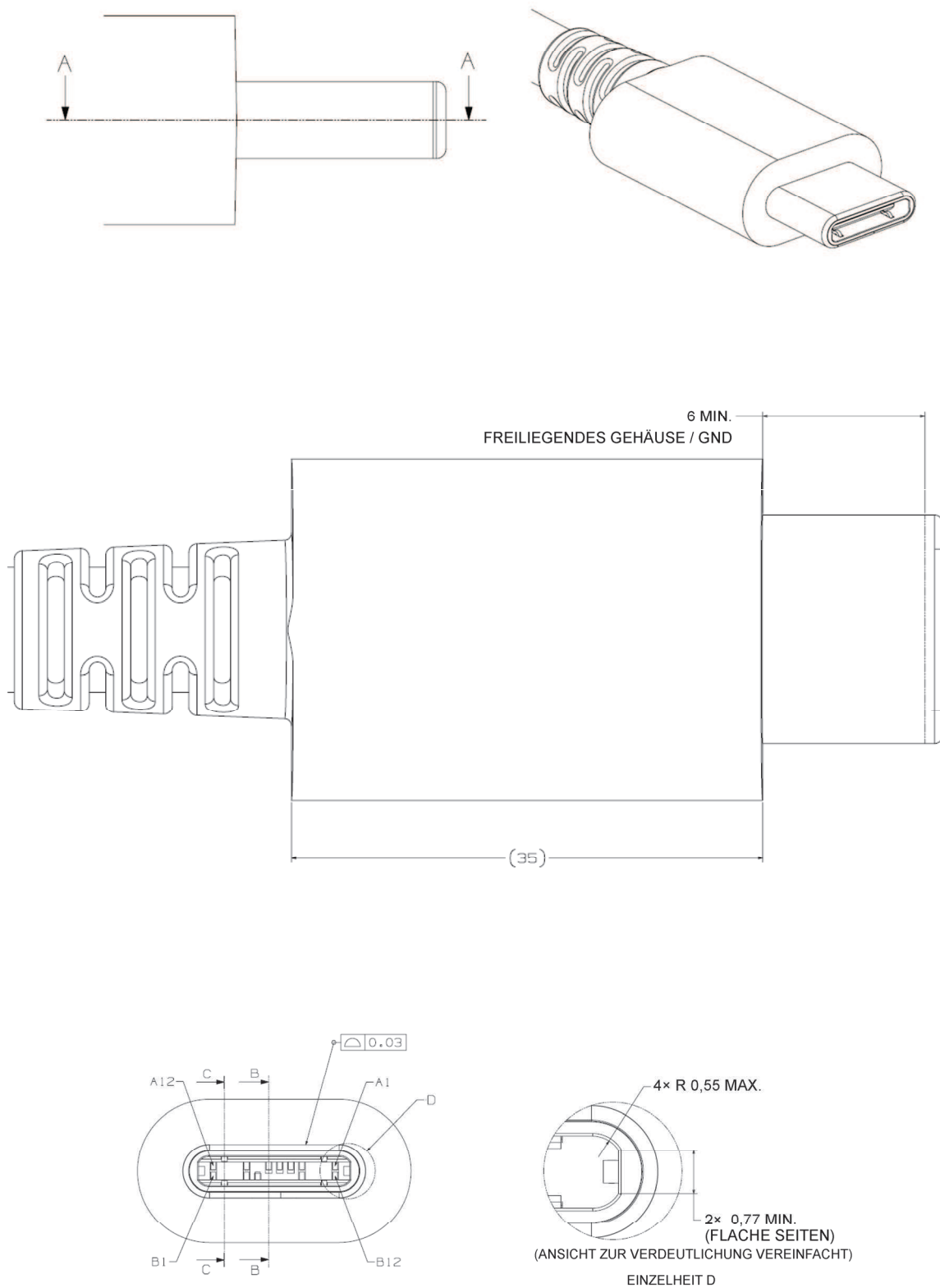
Bild 3-11 – Maße Steckgesicht USB-2.0-Typ-C-Stecker (1 von 3)
