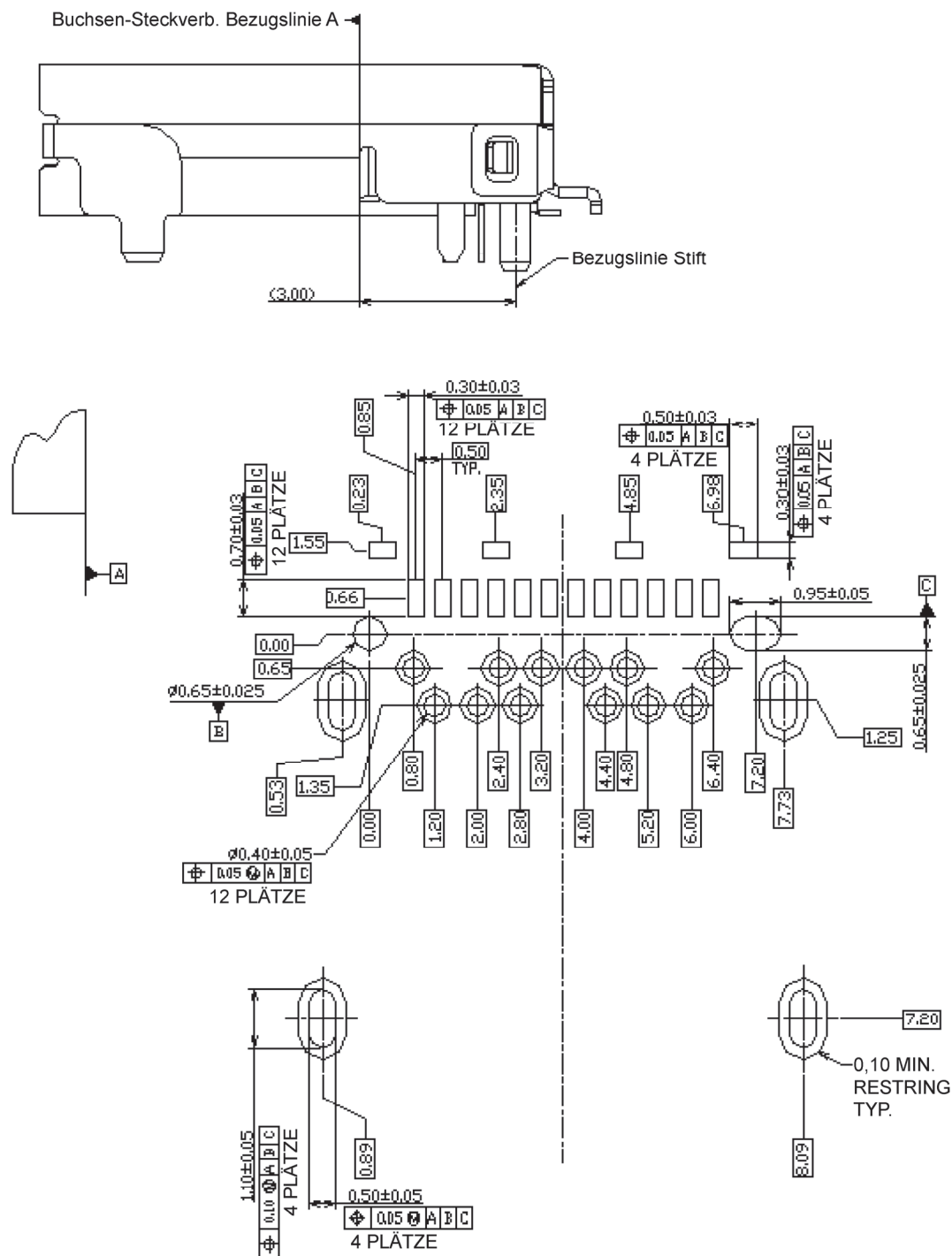
Bild 3-6 – Referenz-Footprint für hybride USB-Typ-C-Buchse mit rechtwinkliger Montage (Informativ)
