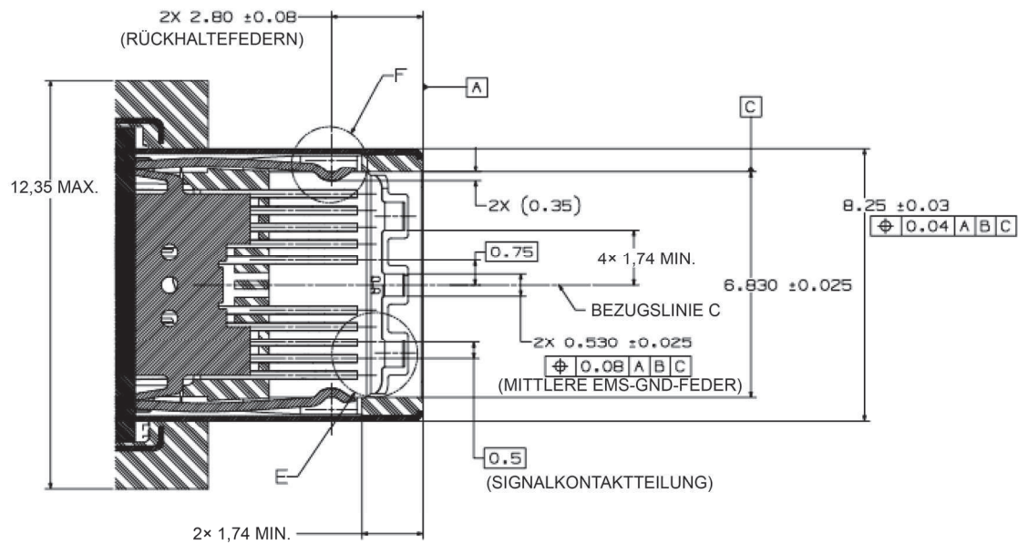
SCHNITT A-A
