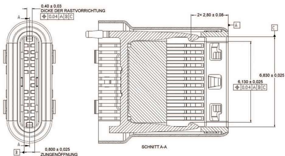
Bild 3-14 – Referenzkonstruktion der Rückhaltevorrichtung
