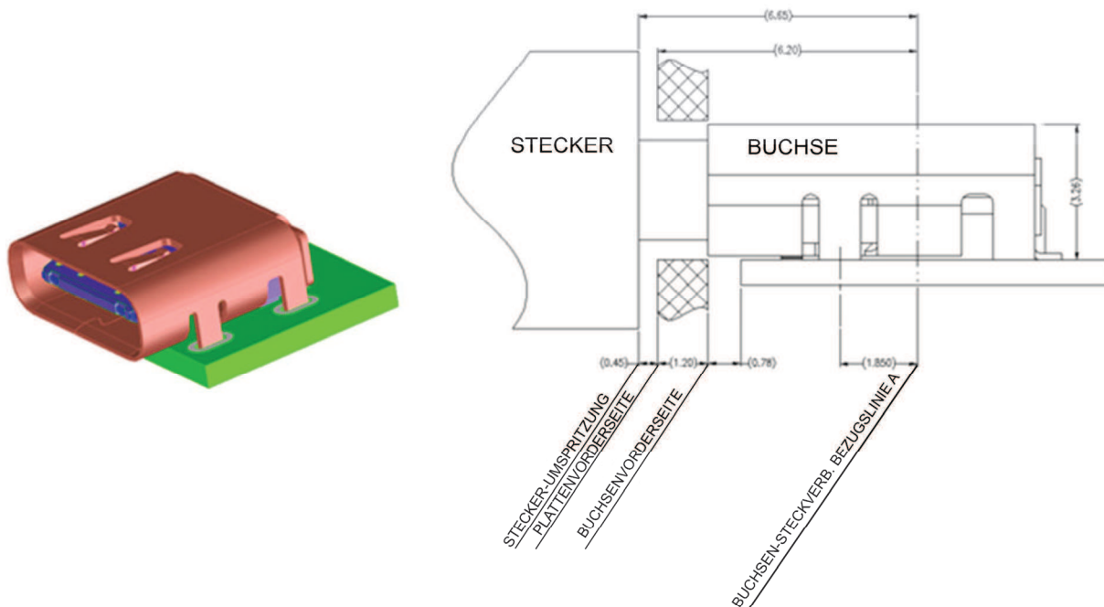
Bild 3-10 – Referenz-Footprint für einreihige USB-2.0-Typ-C-Buchse mit rechtwinkliger Montage (Informativ)
