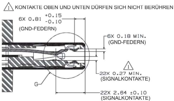
SCHNITT B-B
