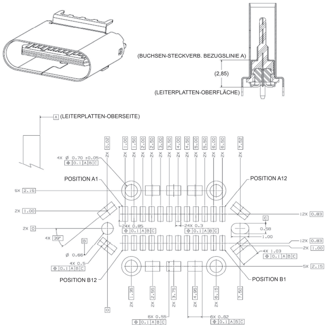
Bild 3-4 – Referenz-Footprint für USB-Typ-C-Buchse mit vertikaler Montage (Informativ)
