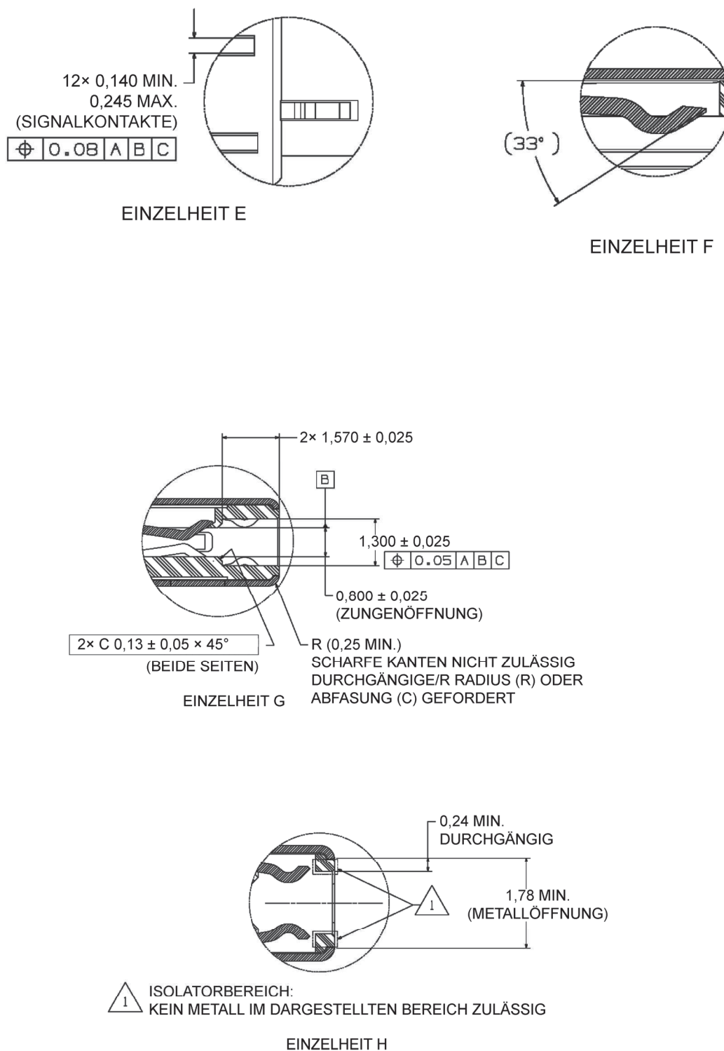
Bild 3-11 – Maße Steckgesicht USB-2.0-Typ-C-Stecker (3 von 3)
