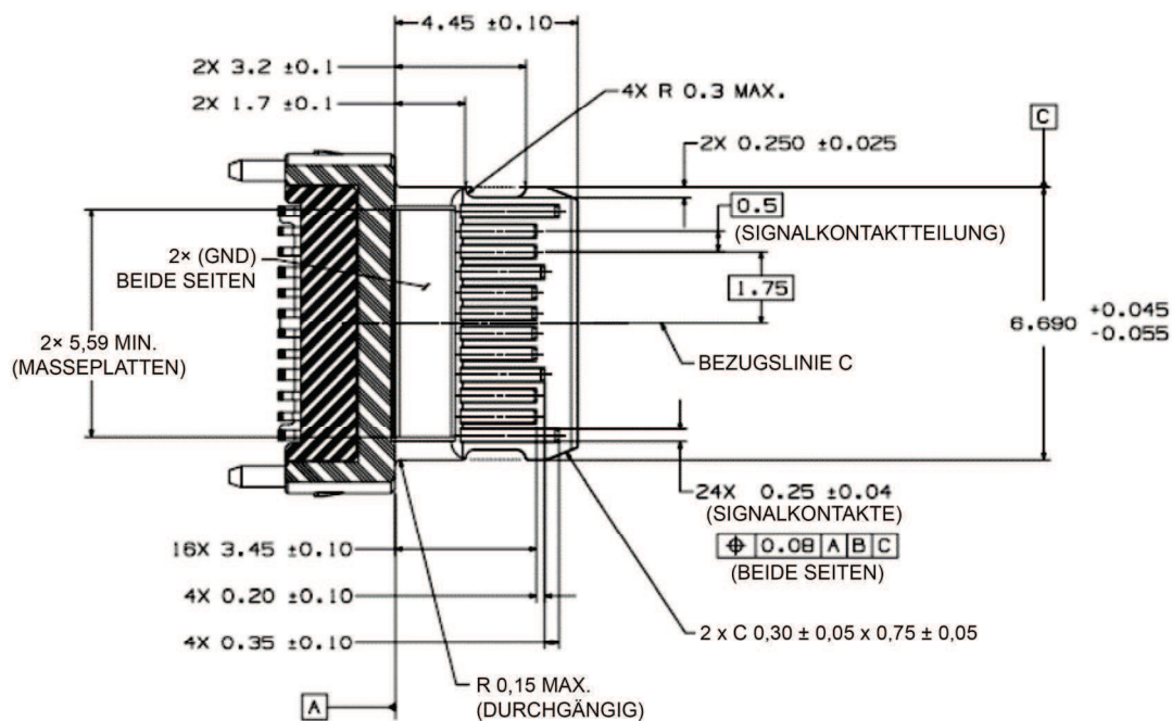
Bild 3-1 – Maße Steckgesicht USB-Typ-C-Buchse (2 von 3)
