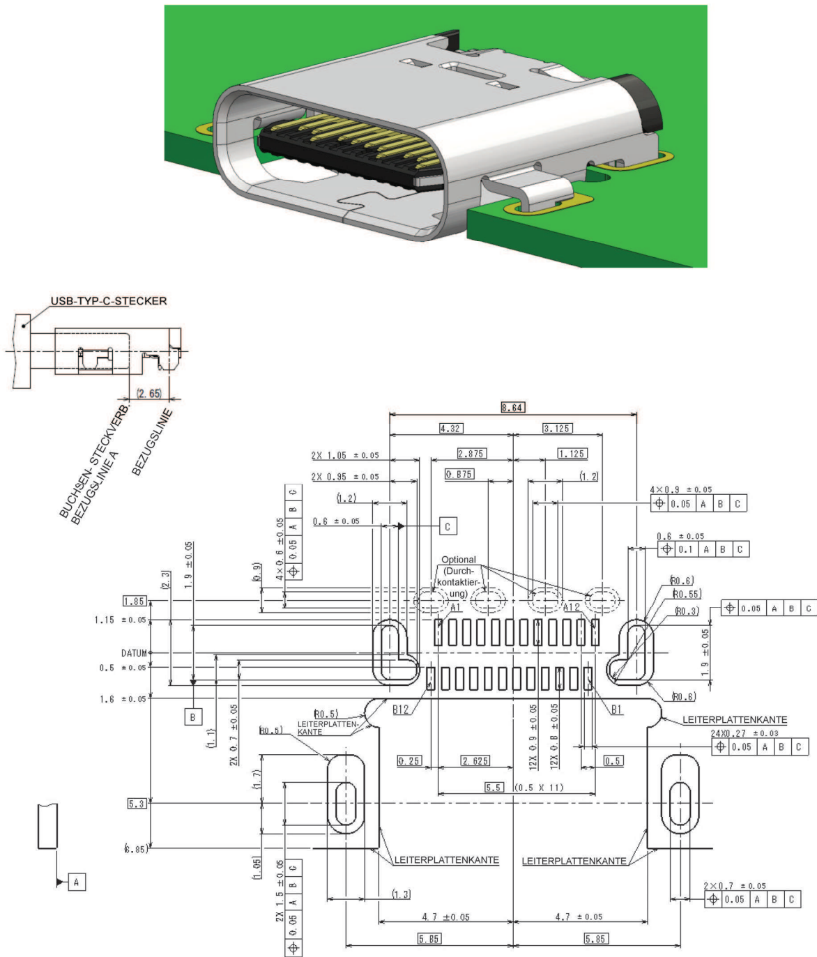
Bild 3-7 – Referenz-Footprint für zweireihige SMT-USB-Typ-C-Buchse mit mittiger Montage (Informativ)
