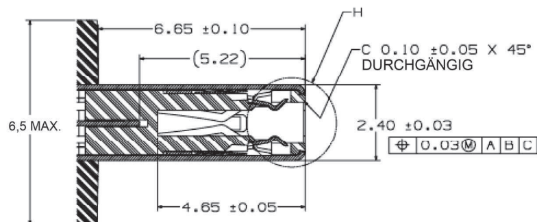
SCHNITT C-C
