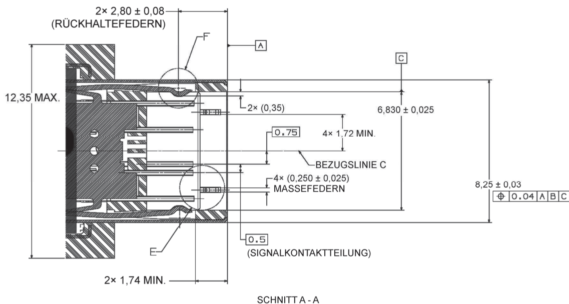
Bild 3-11 – Maße Steckgesicht USB-2.0-Typ-C-Stecker (2 von 3)
