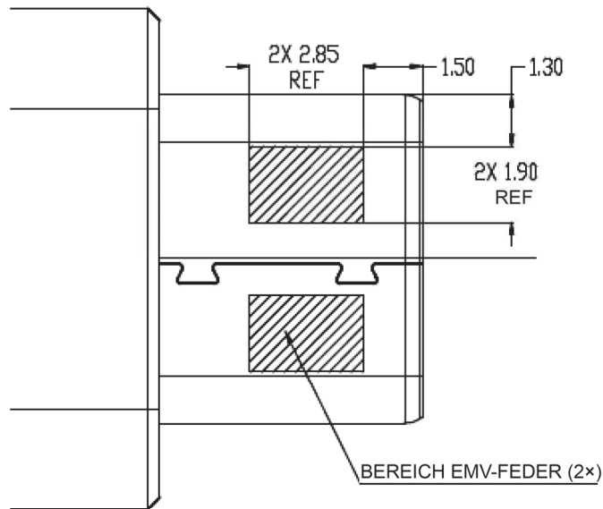
Bild 3-2 – Referenzkonstruktion Kontaktbereiche externe EMV-Feder USB-Typ-C-Stecker
