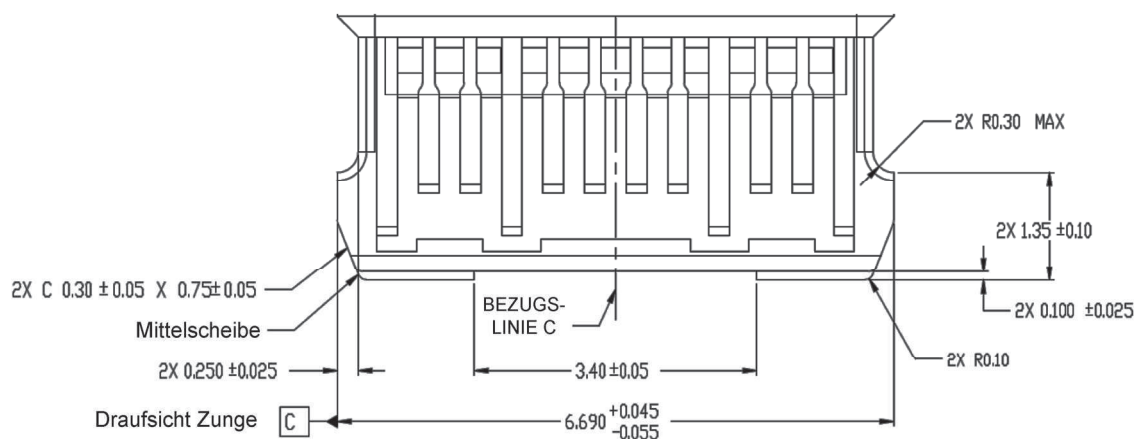
Bild 3-13 – Referenzkonstruktion der Buchsen-Mittelscheibe
