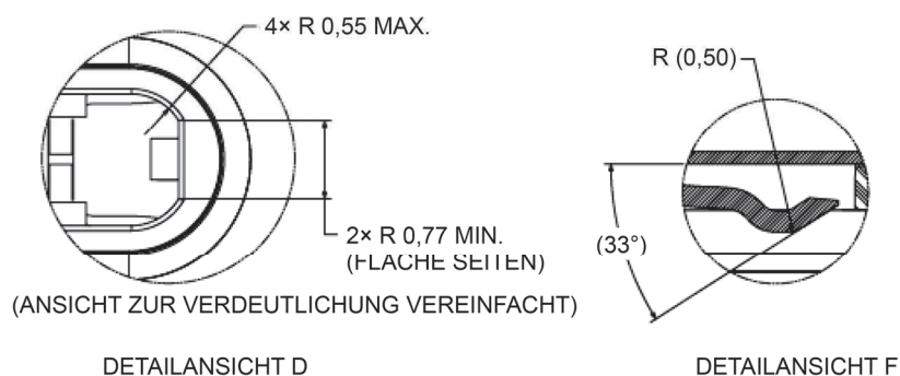
Bild 3-3 – Maße Steckgesicht vollwertiger USB-Typ-C-Stecker (3 von 3)
