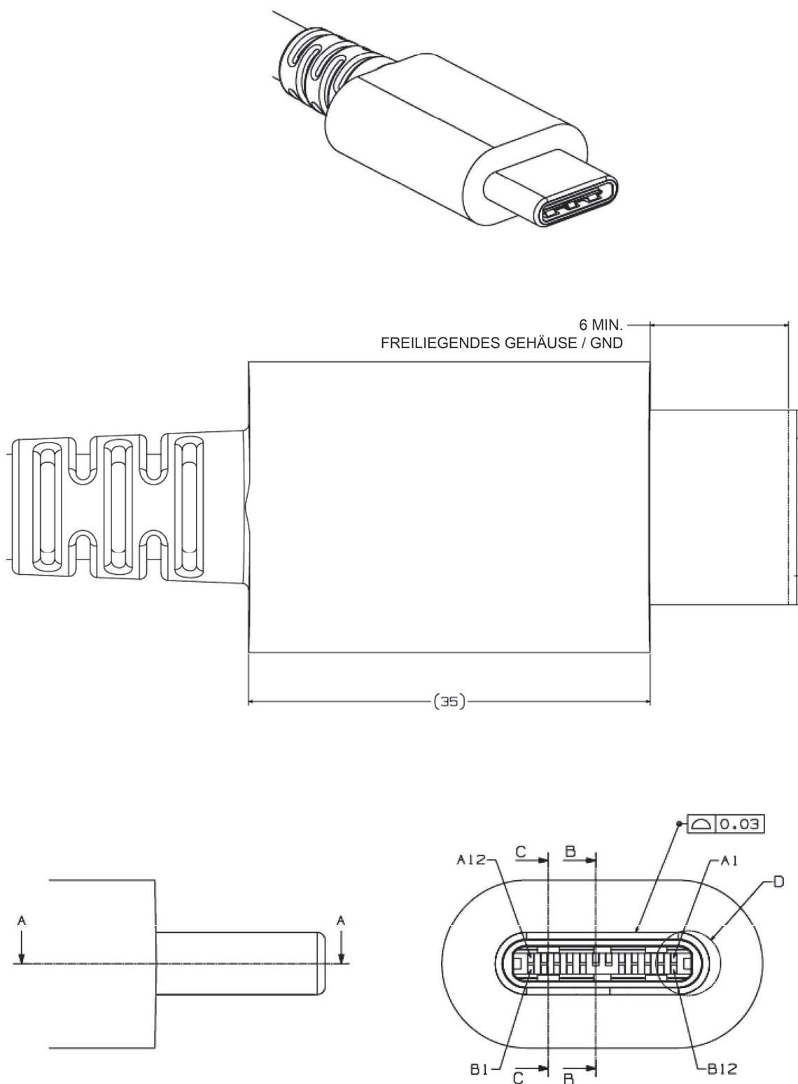
Bild 3-3 – Maße Steckgesicht vollwertiger USB-Typ-C-Stecker (1 von 3)
