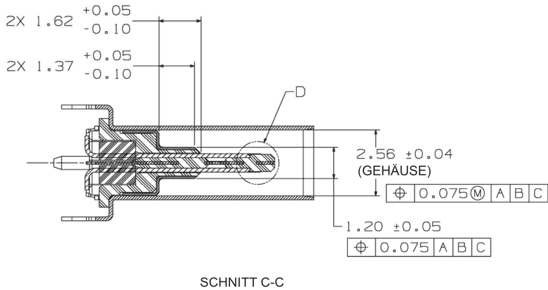
Bild 3-1 – Maße Steckgesicht USB-Typ-C-Buchse (3 von 3)
