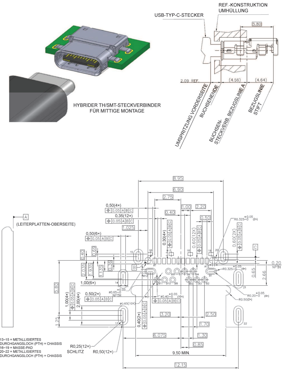
Bild 3-8 – Referenz-Footprint für hybride USB-Typ-C-Buchse mit mittiger Montage (Informativ)
