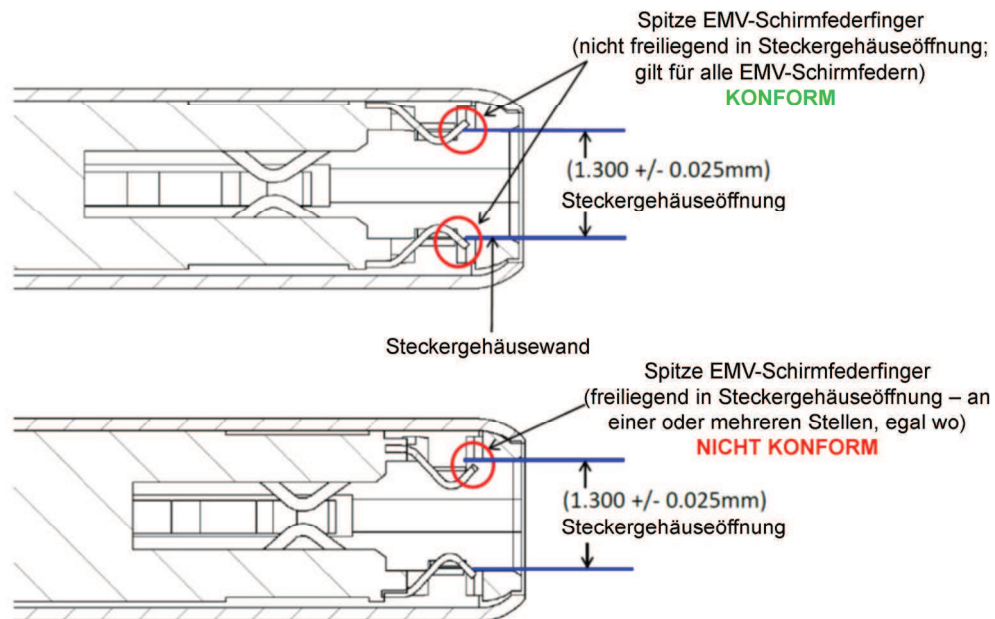
Bild 3-12 – Anforderungen an die EMV-Schirmfederspitzen bei USB-Typ-C-Steckern
