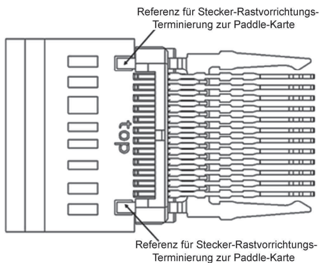
Bild 3-15 – Darstellung der an die Paddle-Karten-Masse gelöteten Rastvorrichtung
