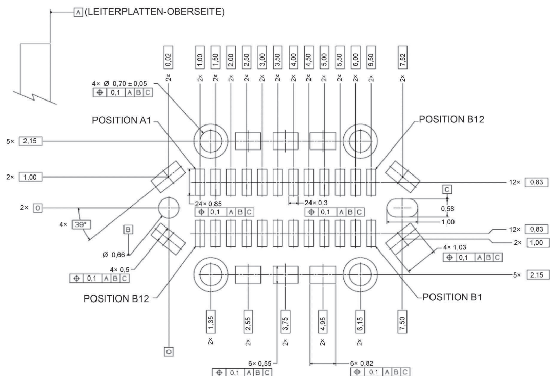
Bild 3-4 – Referenz-Footprint für USB-Typ-C-Buchse mit vertikaler Montage (informativ)
