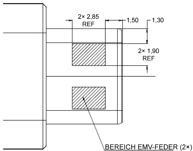
Bild 3-2 – Referenzkonstruktion Kontaktbereiche externe EMV-Feder USB-Typ-C-Stecker
