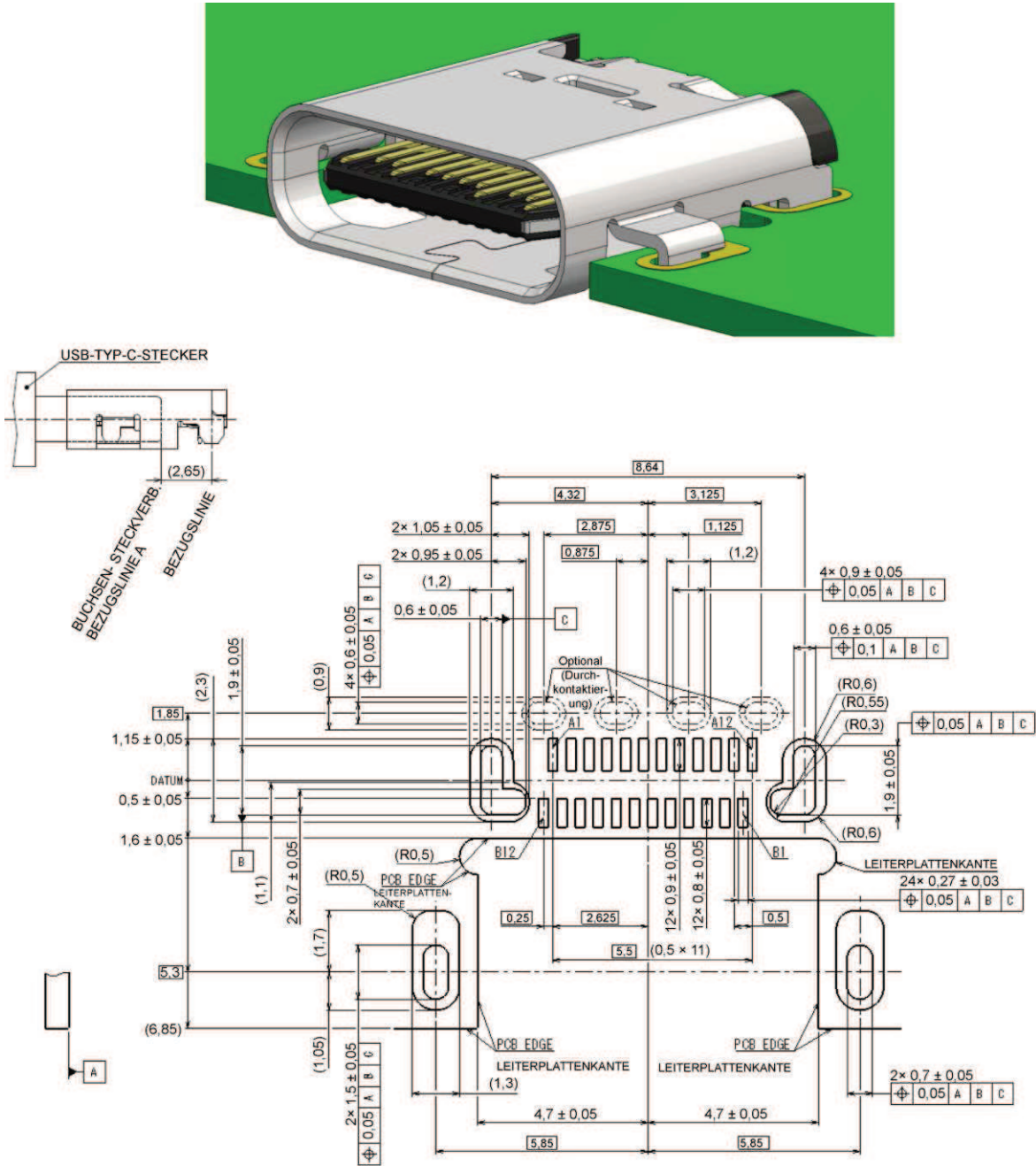
Bild 3-7 – Referenz-Footprint für zweireihige SMT-USB-Typ-C-Buchse mit mittiger Montage (informativ)
