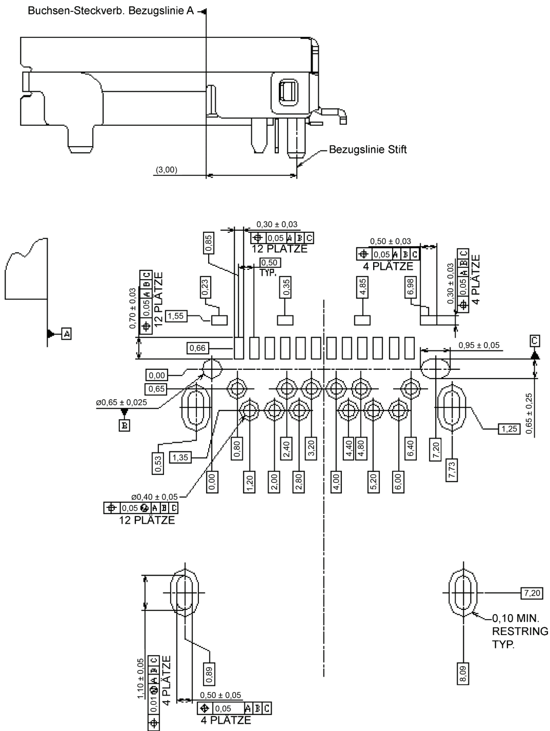
Bild 3-6 – Referenz-Footprint für hybride USB-Type-C-Buchse mit rechtwinkliger Montage (informativ)
