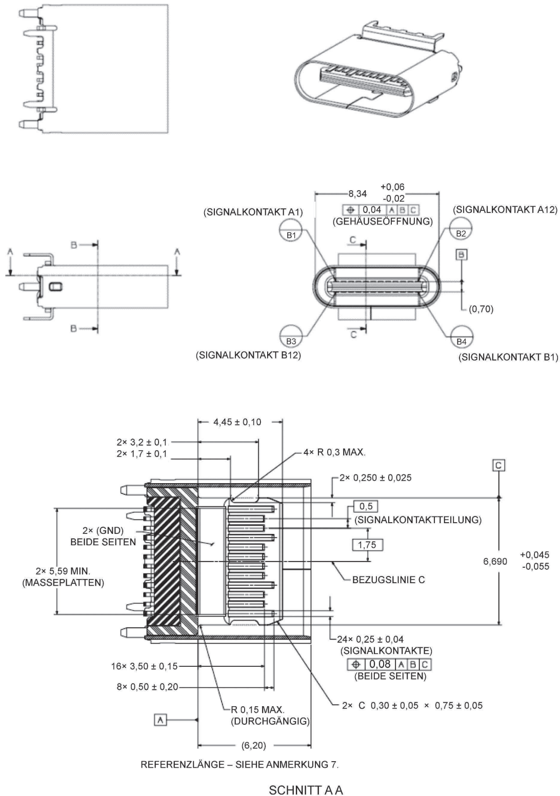
Bild 3-1 – Maße Steckgesicht USB-Typ-C-Buchse
