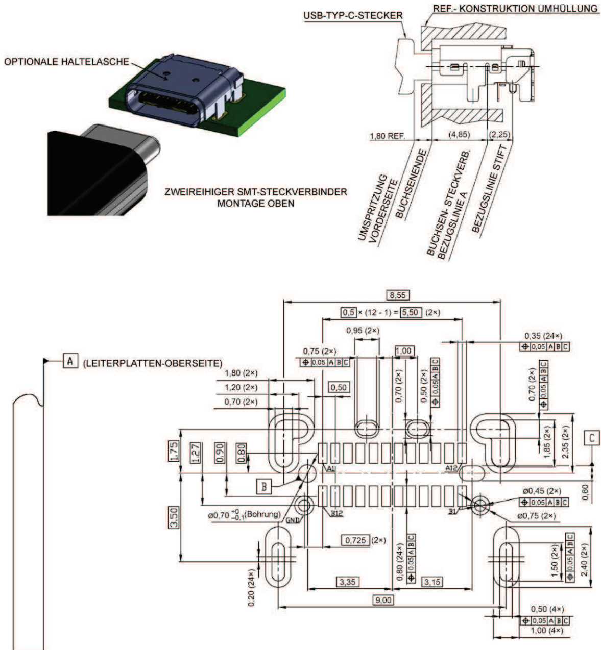
Bild 3-5 – Referenz-Footprint für zweireihige SMT-USB-Type-C-Buchse mit rechtwinkliger Montage (informativ)
