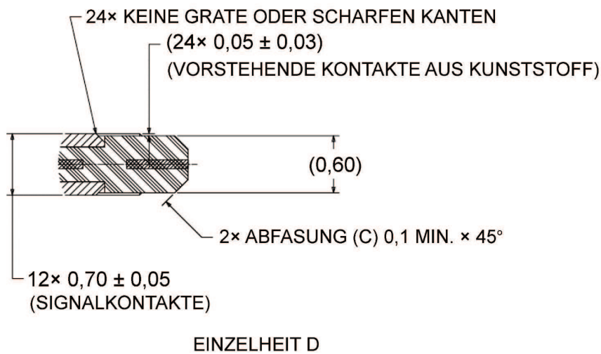
Bild 3-1 – Maße Steckgesicht USB-Typ-C-Buchse, Fortsetzung
