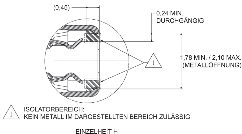
Bild 3-3 – Maße Steckgesicht vollwertiger USB-Typ-C-Stecker, Fortsetzung
