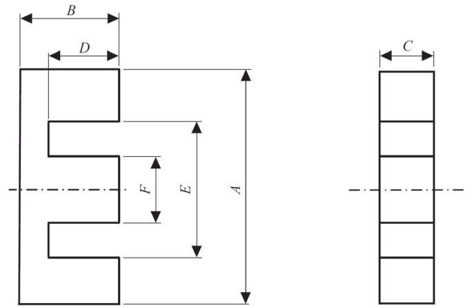
Bild 1 – Maße von E-Kernen mit rechteckigem Querschnitt
