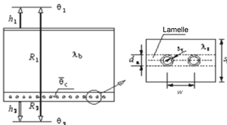
Bild 5 — In eine innenliegende Fläche integrierte Kapillarrohre, Typ F
