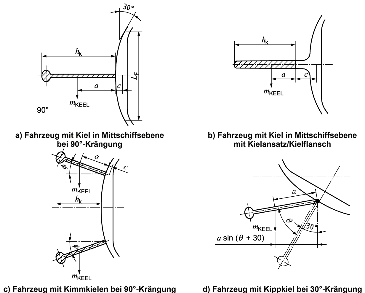
Bild 1 — Skizze von festem Kiel in Mittschiffsebene, Kimmkielen und Kippkiel
