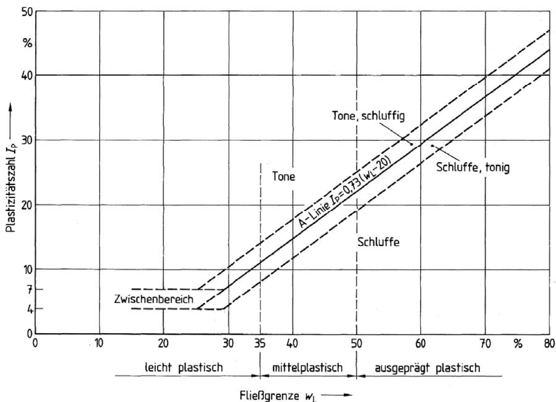
Bild NA.1 — Plastizitätsdiagramm zum Benennen von Bodenarten
