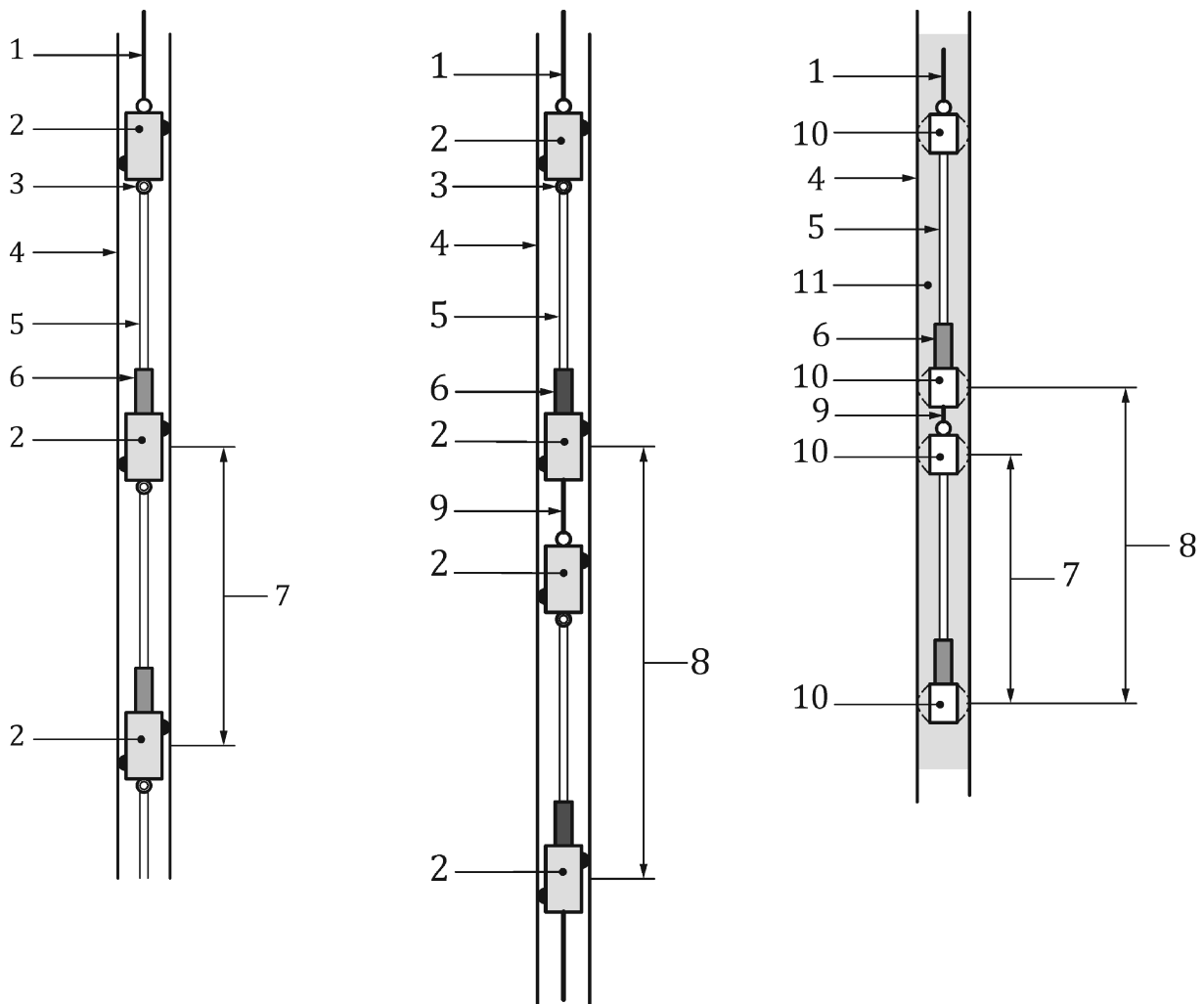
a) IPI mit Rad/Federwippe und kontinuierlicher Kette von Messelementen
