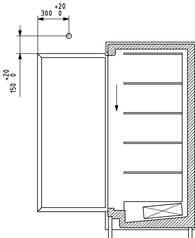
Bild 5 — Klima-Messpunkt für ein typisches Beispiel für ein vertikales Möbel mit Glastüren
