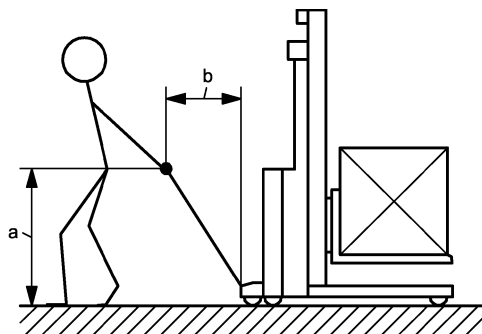
Bild 2 — Deichsel (Schieben)
