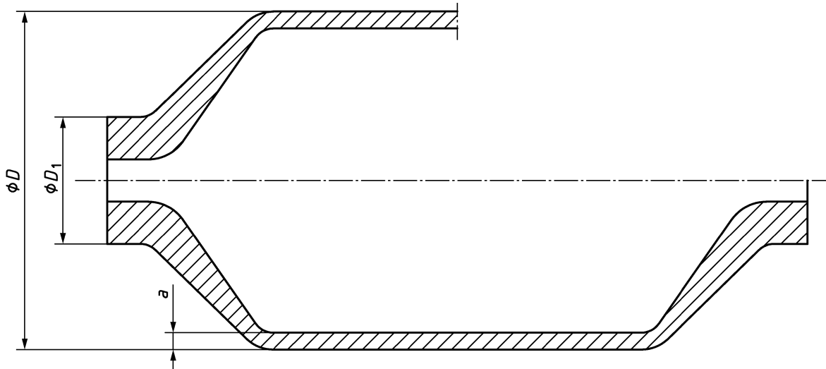
Bild 2 — Rohr-Halsenden
