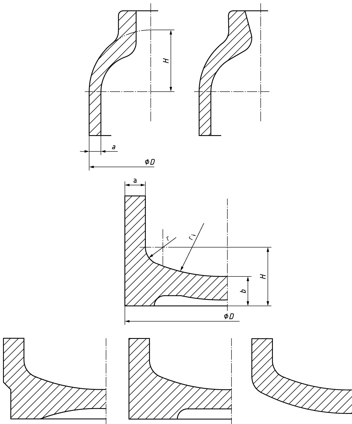
Bild 1 — Typische Ende
