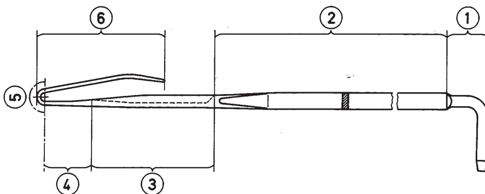
Bild 1. Die Zeichnung zeigt die Hauptteile der Spitzennadel
