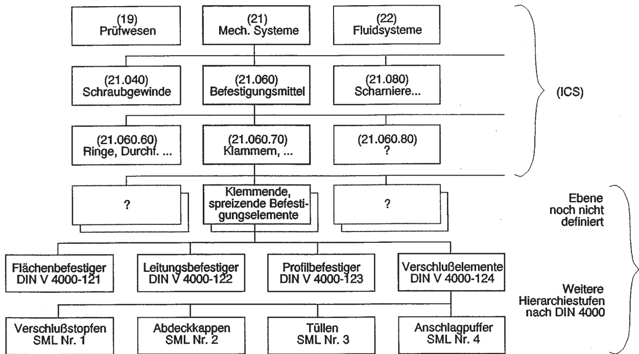
Bild 1: Referenzhierarchie
