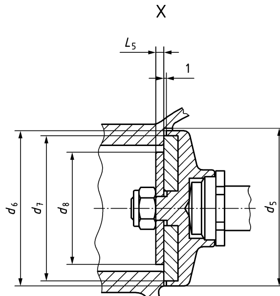
Bild 2 — Detailansicht Ventiltellerdichtung (Detail Z aus Bild 1)
