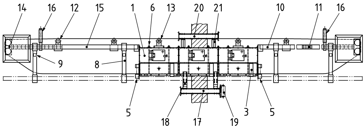
Bild 4 — optional Form B ohne Dichtrahmen (Pos.-Nr 4 und 7) mit Unterbandkasten und Deckelbandkasten
