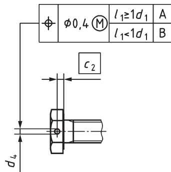
b) Ausführung mit Sicherungsloch
