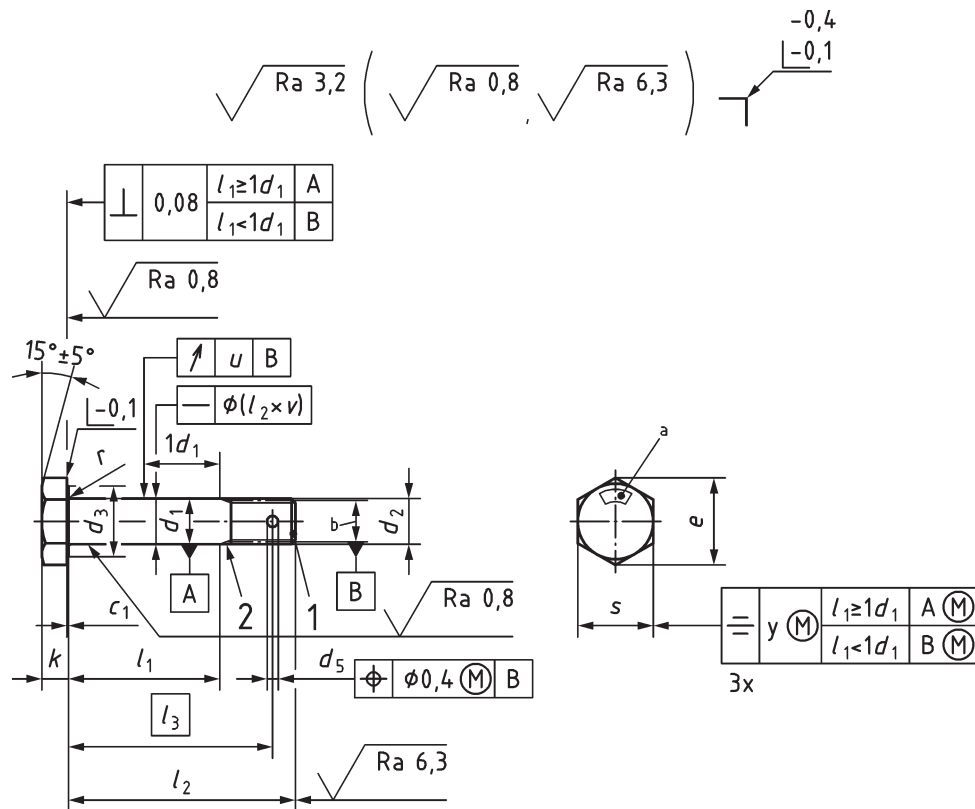
a) Ausführung ohne Sicherungsloch und mit Splintloch
