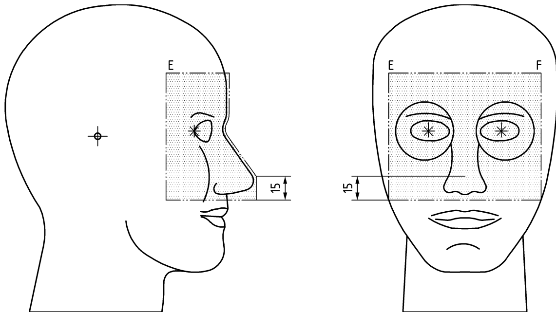
Bild 2 — Schutzbereich (schraffierte Fläche)
