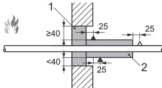
D — Abschottung in einer Aussparung, lokale Rohrisolierung (unterbrochen)
