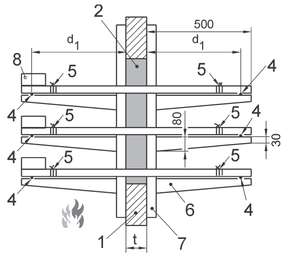
B — Schnitt A-A
