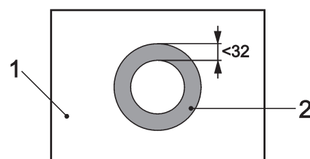
E — Lage der Thermoelemente an herausragenden Teilen der Abschottung
