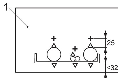
D — Lage der Thermoelemente in Bezug auf Kabel und Kabeltrassen
