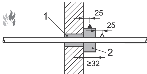
C — Abschottung mit zusätzlicher Komponente. Beispiele: Rohrmanschette oder Kabelschutz mit z. B. einer Bandage aus Mineralwolle
