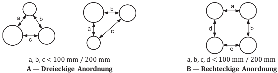
Bild 4 — Gruppenanordnung von Abschottungen/Leitungen
