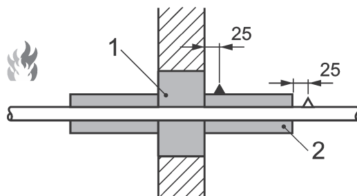
F — Lokale Rohrisolierung (unterbrochen)
