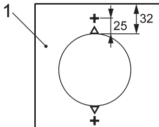
A — Lage der Thermoelemente in Bezug auf kleine Rohre/andere Leitungen (Umfang \leq 500 mm oder Durchmesser \leq 160 mm bei runden Leitungen)
