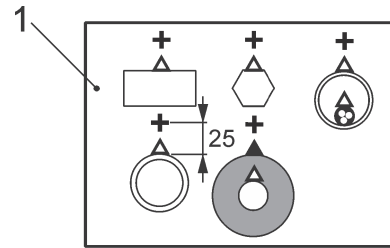
B — Lage der Thermoelemente in Bezug auf große Rohre/andere Leitungen (Umfang > 500 mm oder Durchmesser > 160 mm bei runden Leitungen)
