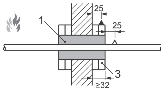
H — Einsatz einer Aufleistung (z. B. aus Gipsplattenstreifen) zum Abstützen der Abschottung, Dicke der Aufleistung ≥ 32 mm
