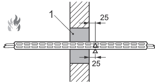
B — Thermoelement-Position A auf Kabeltragekonstruktion nach 9.1.2.2
