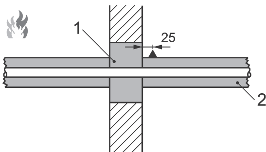
E — Durchgehende Rohrisolierung (unterbrochen)
