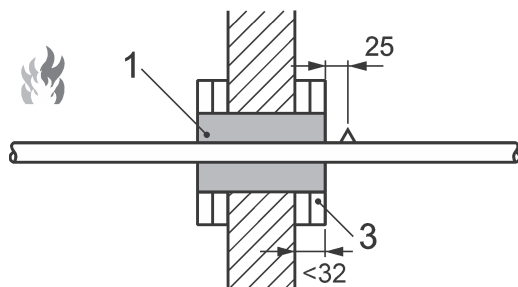
G — Einsatz einer Aufleistung (z. B. aus Gipsplattenstreifen) zum Abstützen der Abschottung, Dicke der Aufleistung < 32 mm
