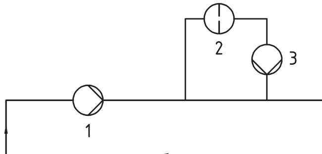
Bild 3 — Dynamisches Spülen in der Hauptzirkulation
