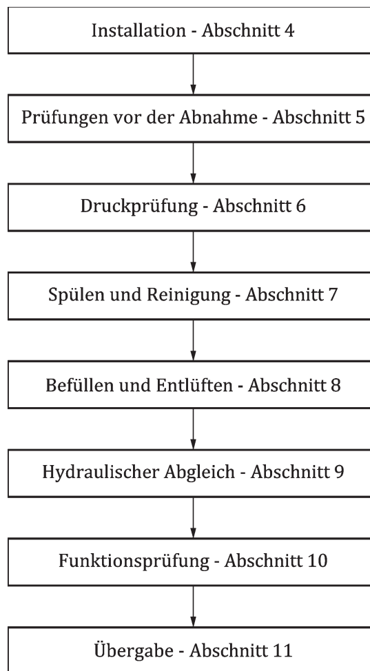
Bild 1 — Aufbau- und Abnahmeverfahren
