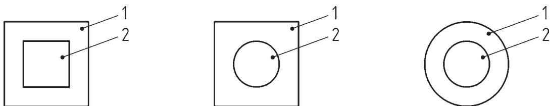
a) Konzentrische Luft/Abgas-Anordnungen
