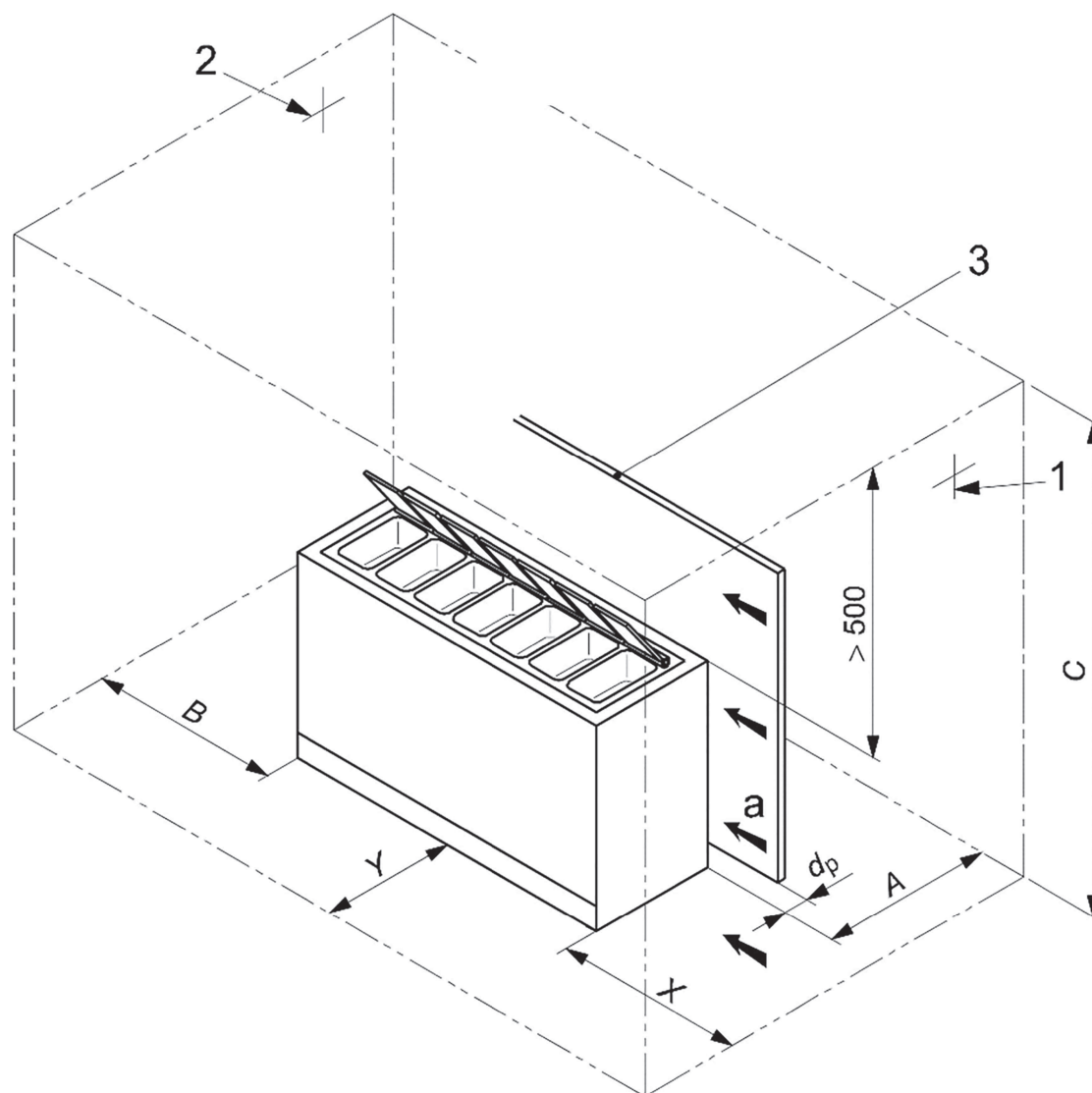
b) Position des Verkaufskühlmöbels für Speiseeis, Beispiel 2
