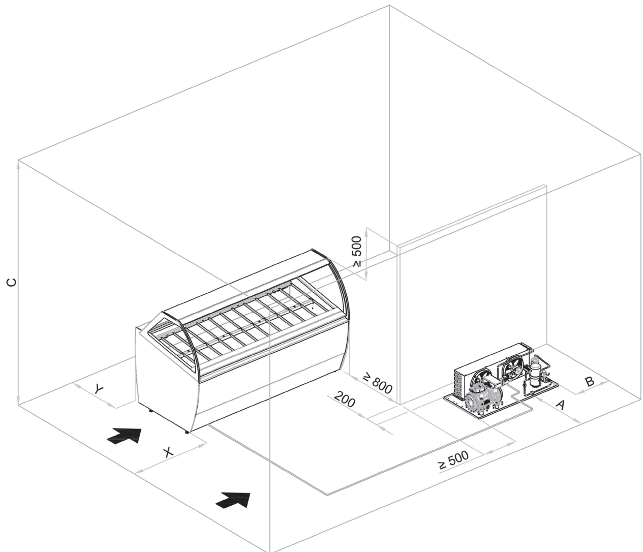
a) Position des Verkaufskühlmöbels für Speiseeis und seines eigenen Split-Verflüssigungssatzes
