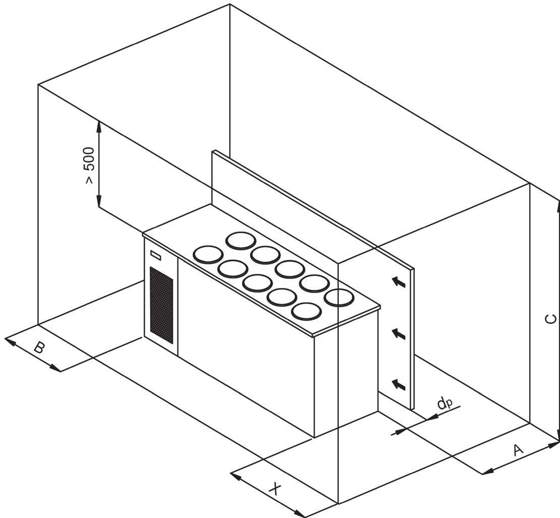
c) Position des Pozzetto für Speiseeis
