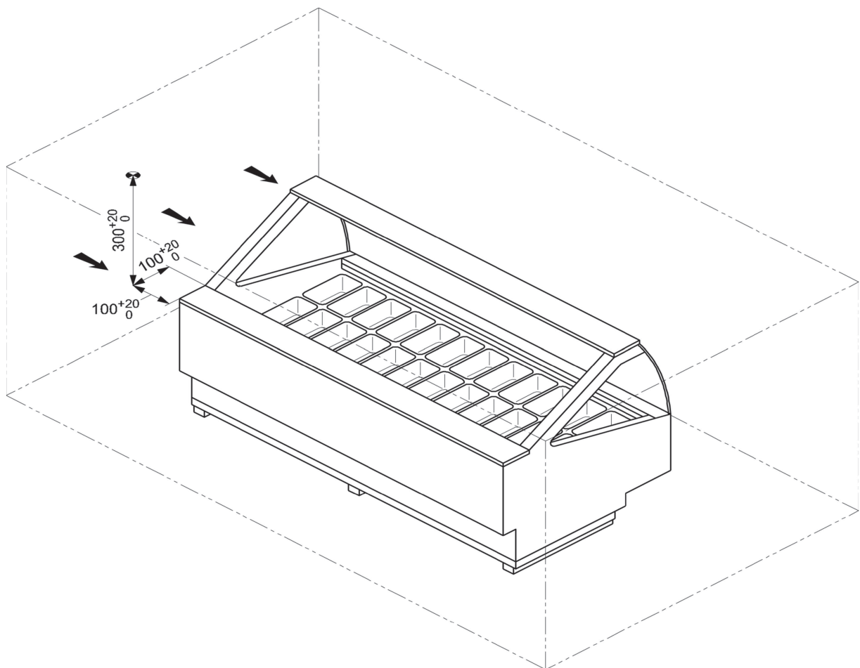
a) Position des Verkaufskühlmöbels für Speiseeis, Beispiel 1
