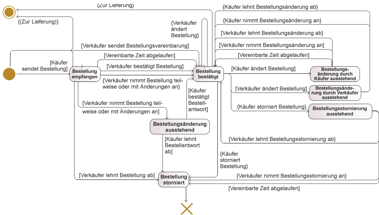
Bild 3 — Maschinen-Bestellzustandsdiagramm [informativ]
