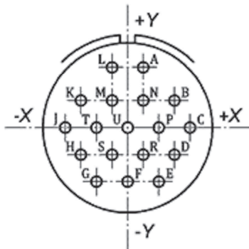
15N18 Klasse I 18 Kontakte, Größe 20
