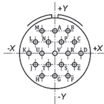
15N19 Klasse I 19 Kontakte, Größe 20
