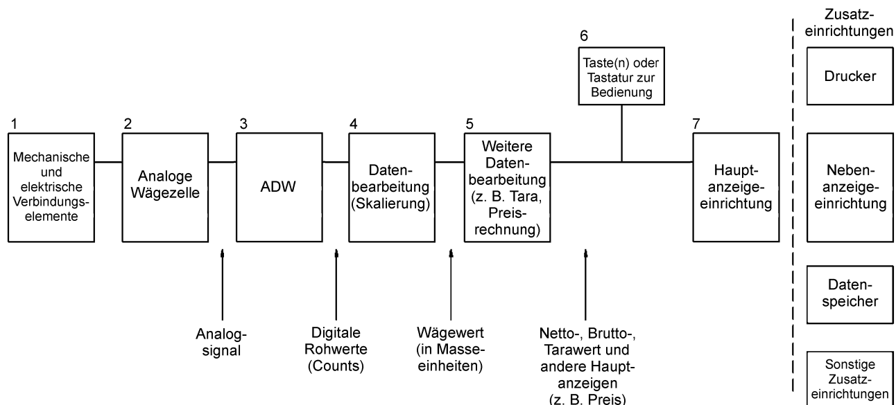
Bild 1 — Definition typischer Module nach T.2.2 und 3.10.2 (andere Kombinationen sind möglich)
