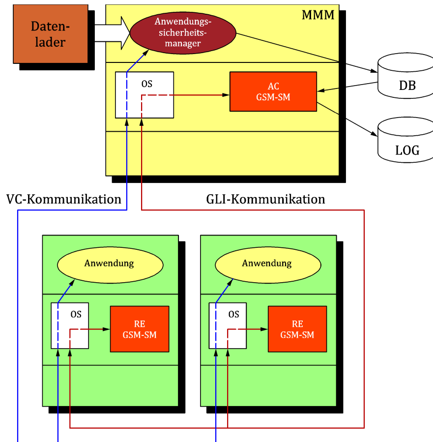
Bild 24 — Wesentliche sicherheitsbezogene Architekturkomponenten
