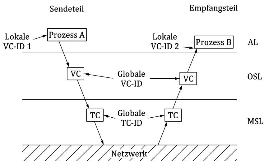
Bild 13 — Kommunikationskonzept
