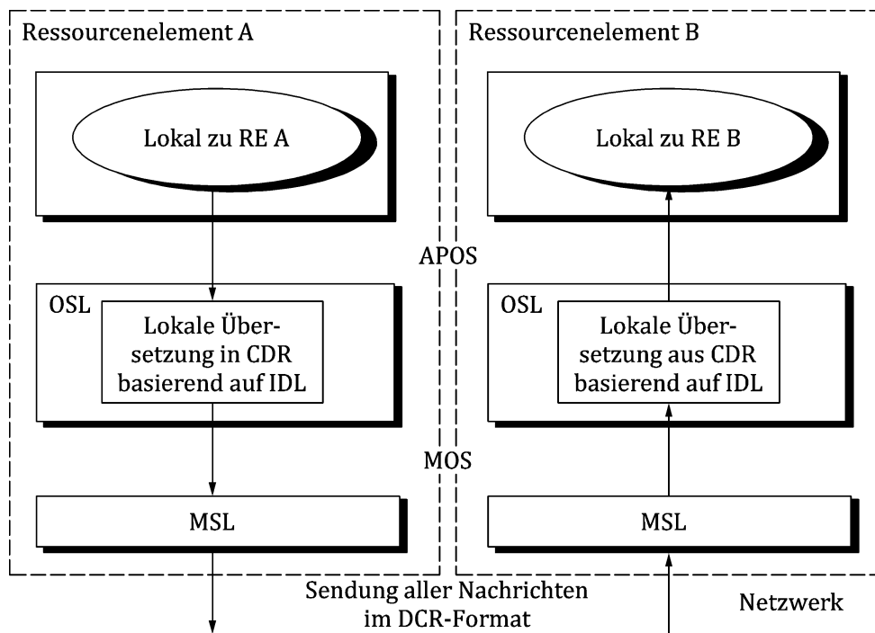
Bild 22 — Datendarstellung
