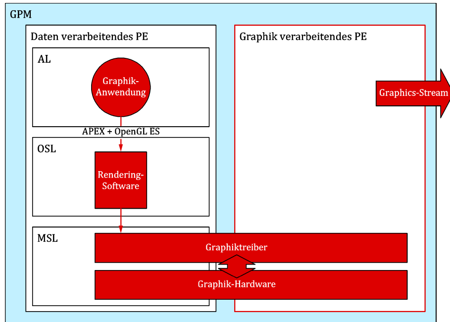
Bild 28 — MOAA-Graphikarchitektur
