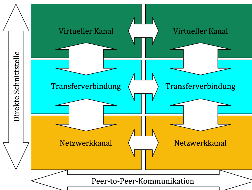
Bild 9 — Der MOAA-Kommunikationsstapel
