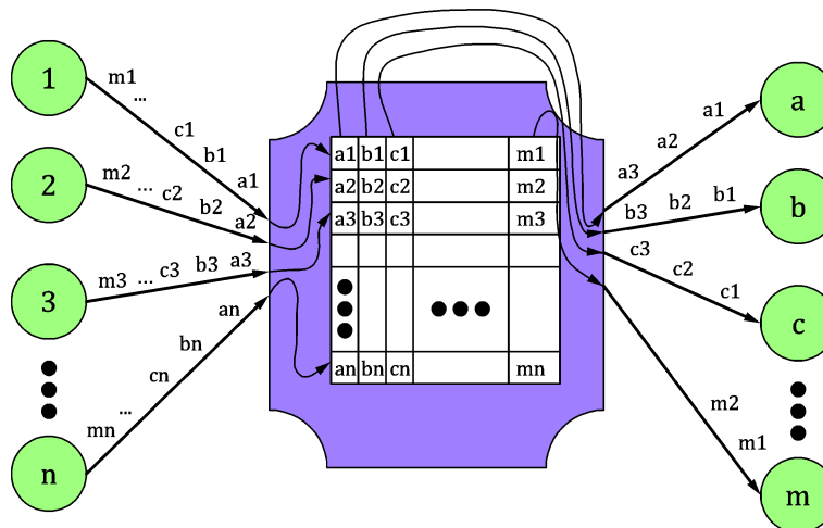
Bild 19 — Corner-Turn
