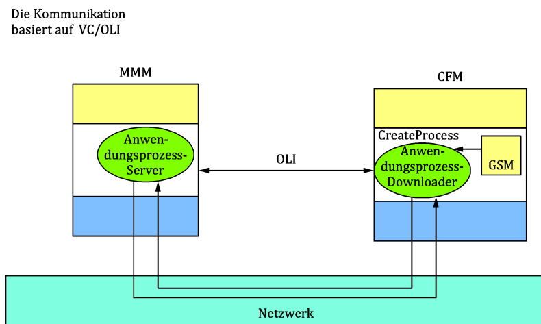
Bild 27 — Anwendungsdownload
