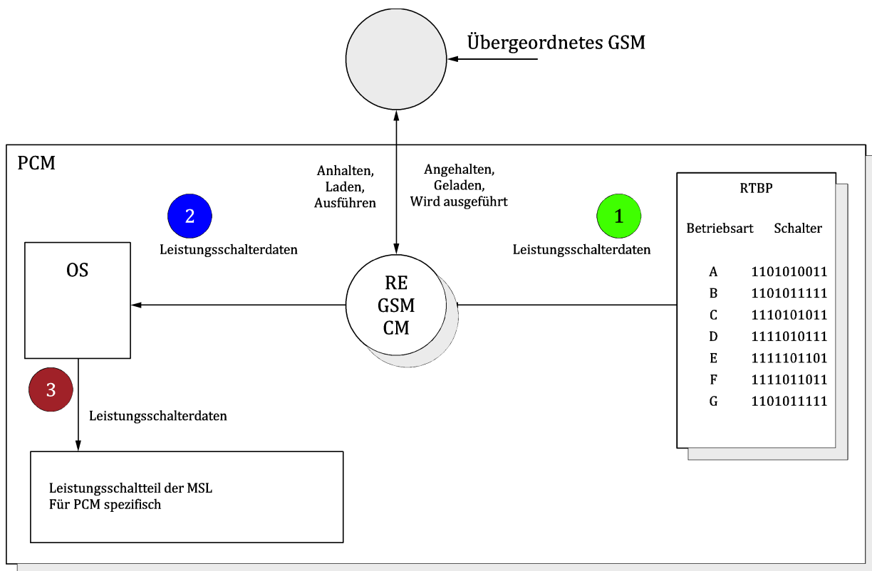
Bild 29 — PCM-Verwaltung (Beispiel)
