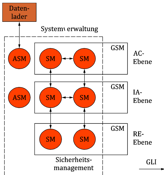
Bild 23 — GSM-Schnittstellen
