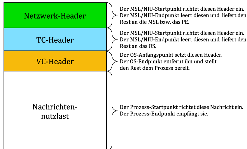
Bild 15 — MOAA-Nachricht bei BMC-Datentransfer
