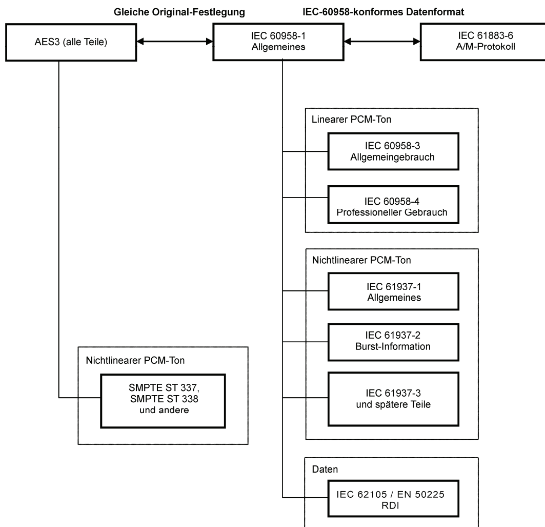
Bild C.1 – Zusammenhang der IEC-60958-Familie
