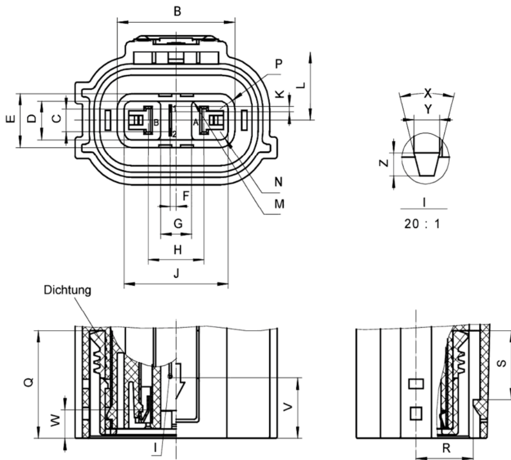
Bild 6 – 2-poliger freier 40 A-Steckverbinder
