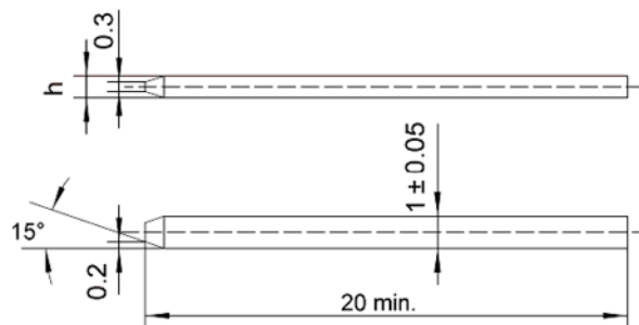
Bild 9 – Lehre für Signalkontakt
