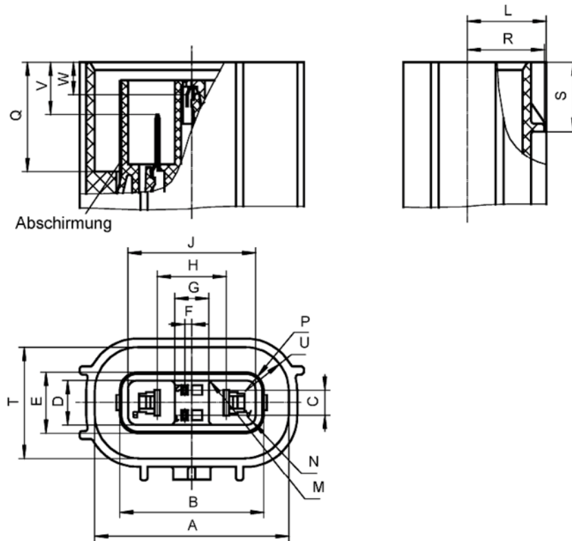
Bild 3 – 2-poliger fester 40 A-Steckverbinder
