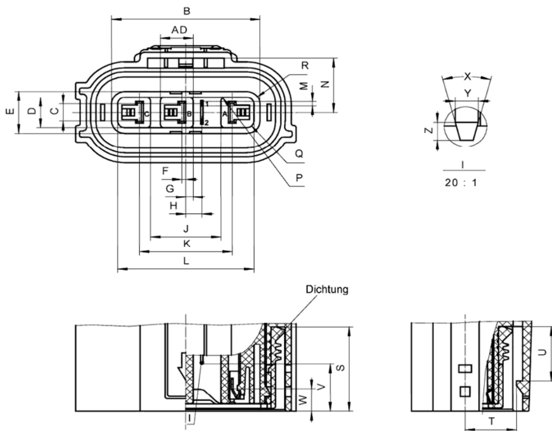
Bild 7 – 3-poliger freier 40 A-Steckverbinder
