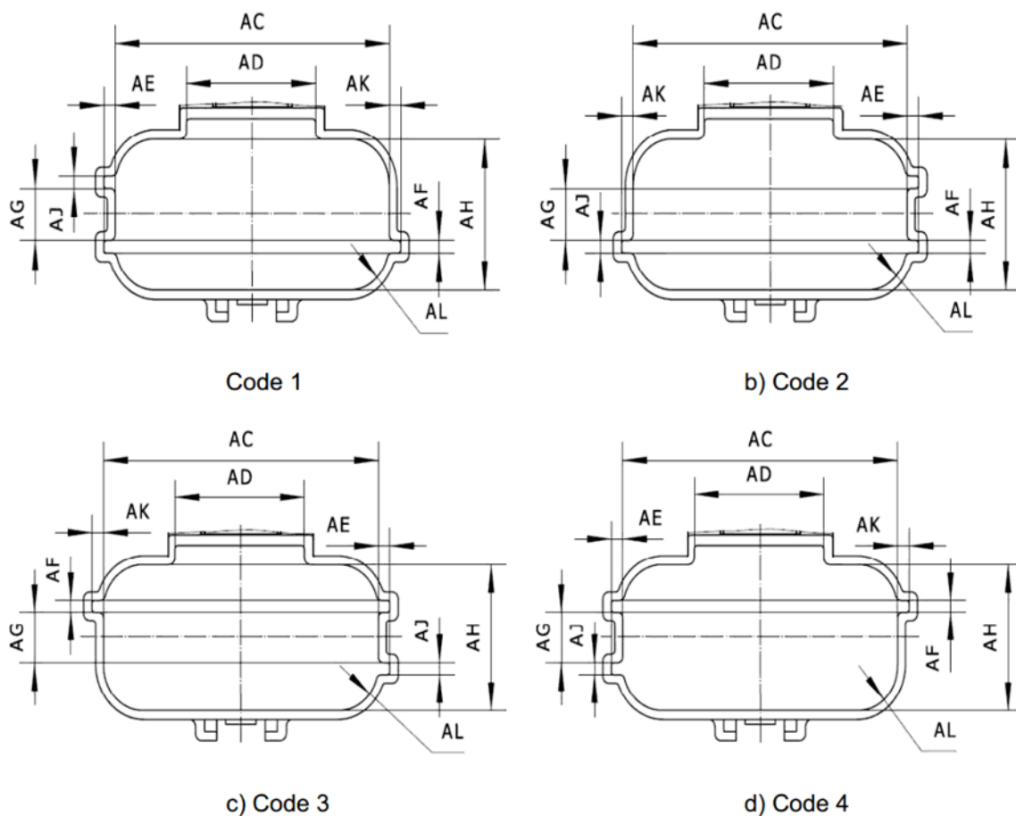
Bild 8 – Codes freier Steckverbinder
