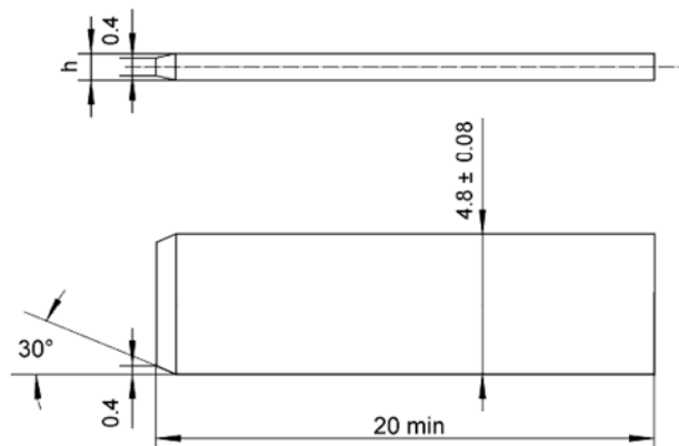
Bild 10 – Lehre für Leistungskontakt
