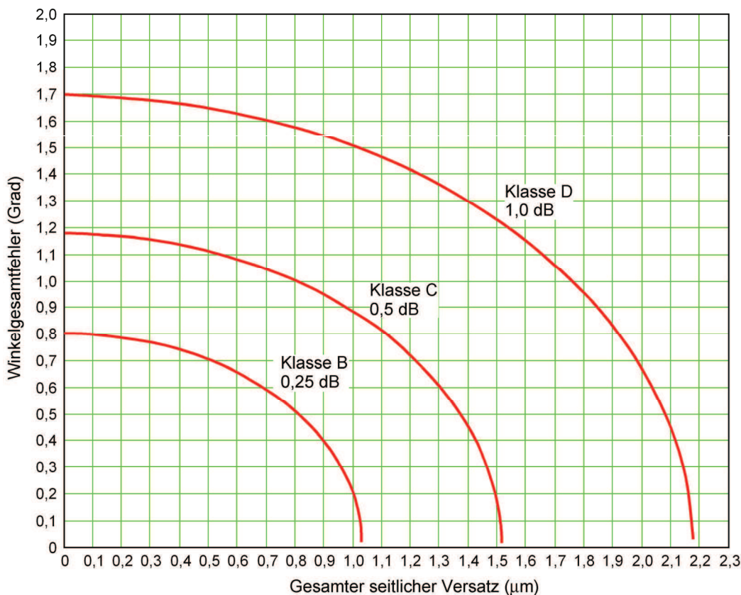
Bild 1 – Seitlicher Versatz und Winkelversatz in Abhängigkeit von der Dämpfung \eta_{\text{kombiniert}} für Einmodenfasern mit 8,9 µm MFD
