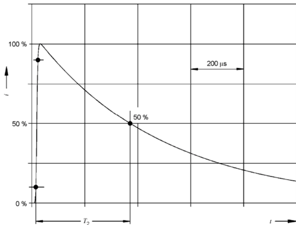
Bild B.2 – Zeitlicher Verlauf des Rückens des ersten positiven Stoßstroms
