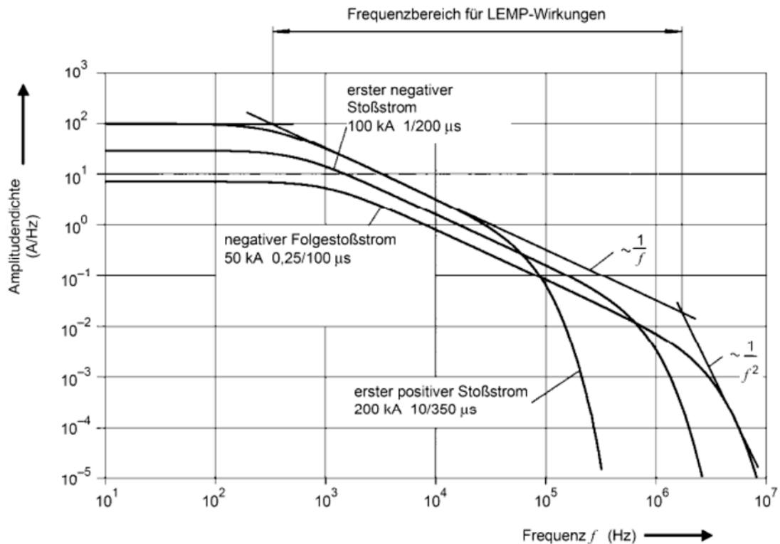
Bild B.7 – Amplitudendichte des Blitzstroms entsprechend Gefährdungspegel LPL I
