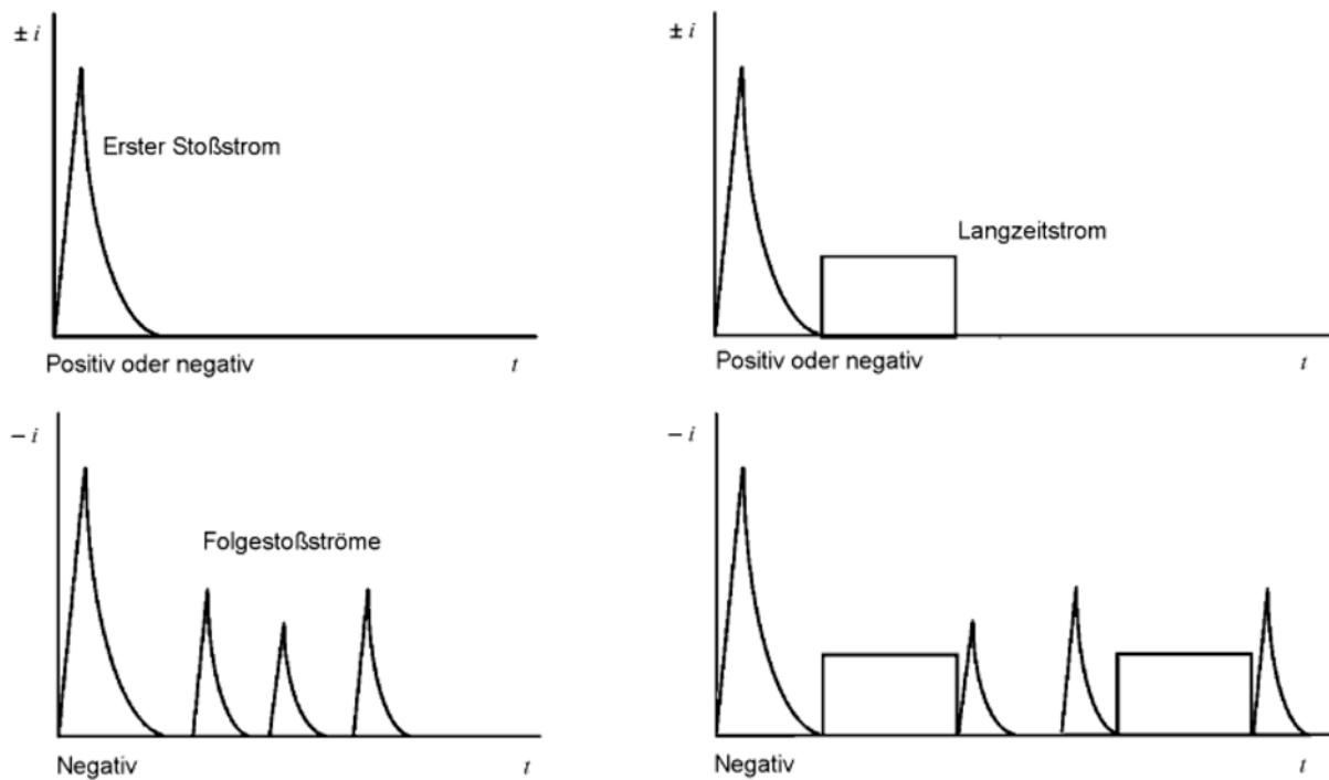
Bild A.3 – Mögliche Komponenten von Abwärtsblitzen (typisch in flacher Umgebung und für niedrige bauliche Anlagen)
