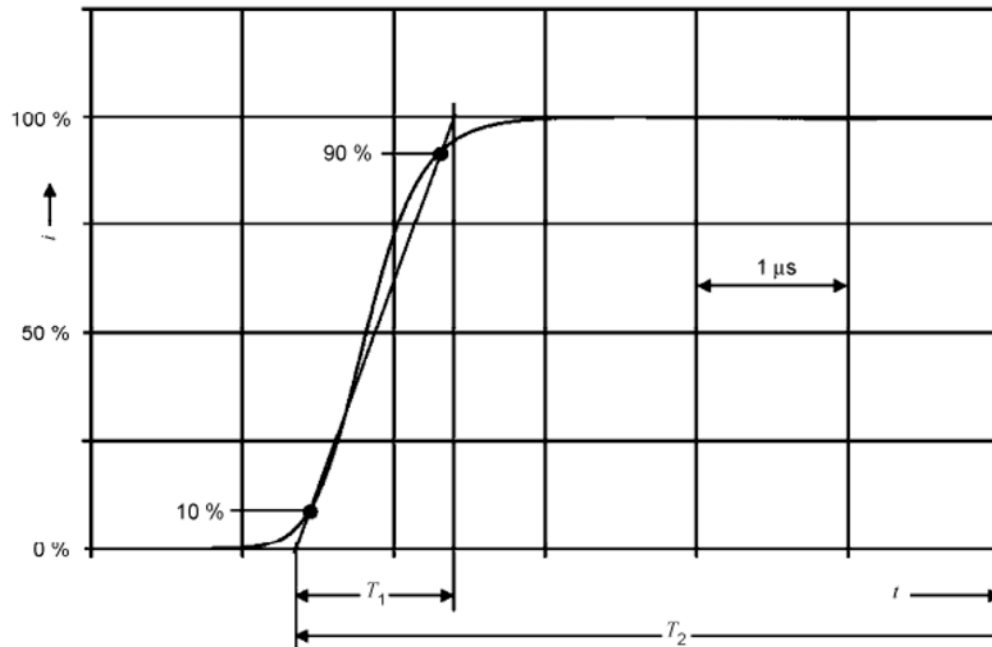
Bild B.3 – Zeitlicher Verlauf der Stirn des ersten negativen Stoßstroms
