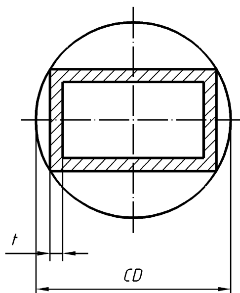
Bild 2 — Umschlingungskreis für Rohre, ausgenommen Rundrohre
