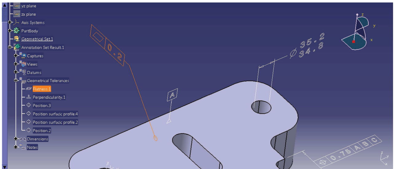
Bild 5 — Veranschaulichung der PMI-Konvertierung als Linienzugpräsentation (STEP-Export und -Import)
