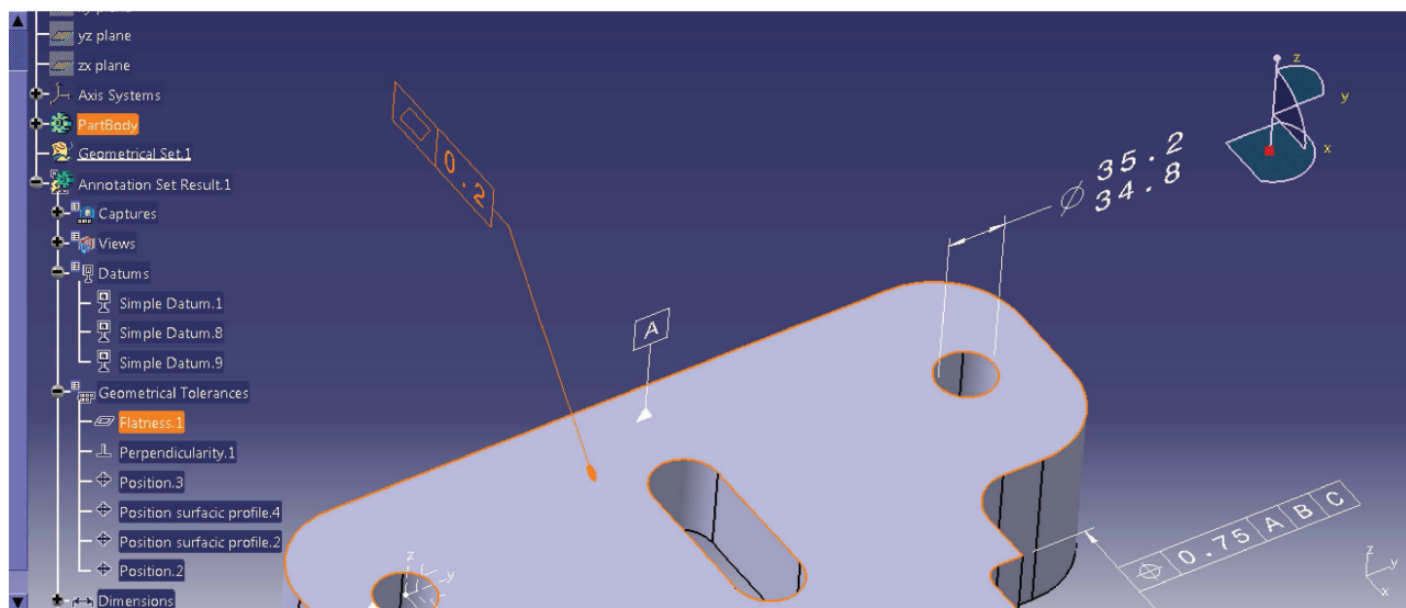
Bild 7 — Veranschaulichung der PMI-Konvertierung als tesselierte Darstellung (STEP-Export und -Import)
