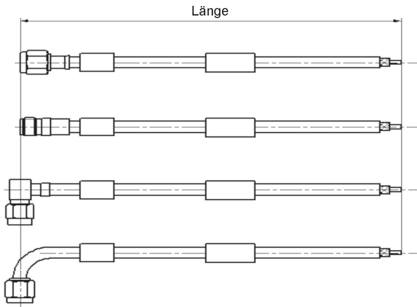
Bild 2 – Definition der Länge von konfektionierten Kabeln mit einem Steckverbinder
