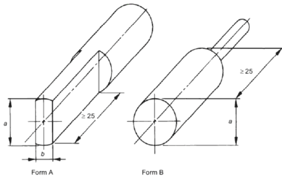
Bild 26 – Prüflehren Form A und Form B
