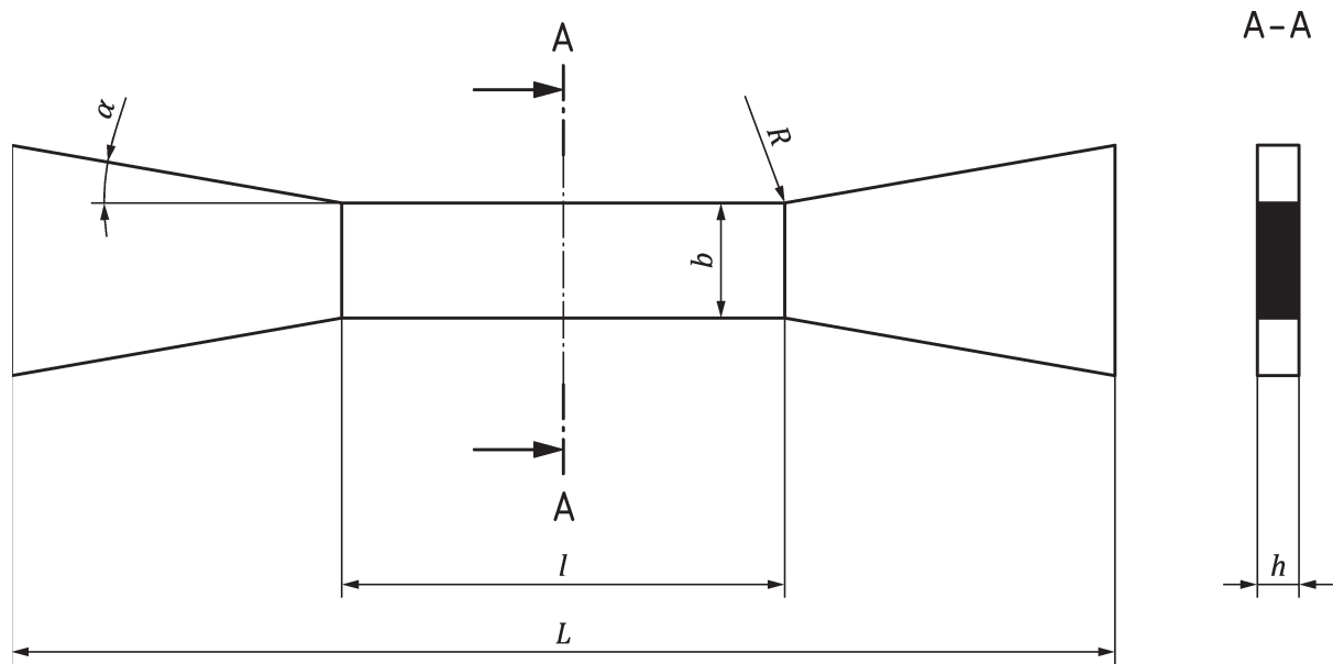
Bild 1 — Probekörper vom Typ 1
