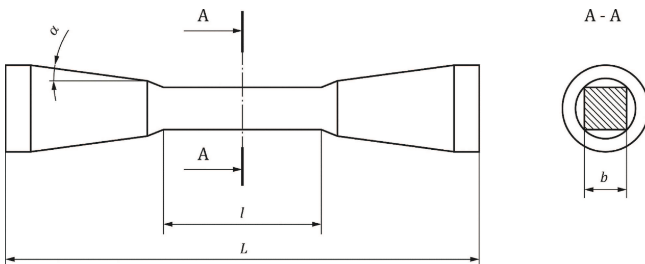
Bild 3 — Probekörper vom Typ 3
