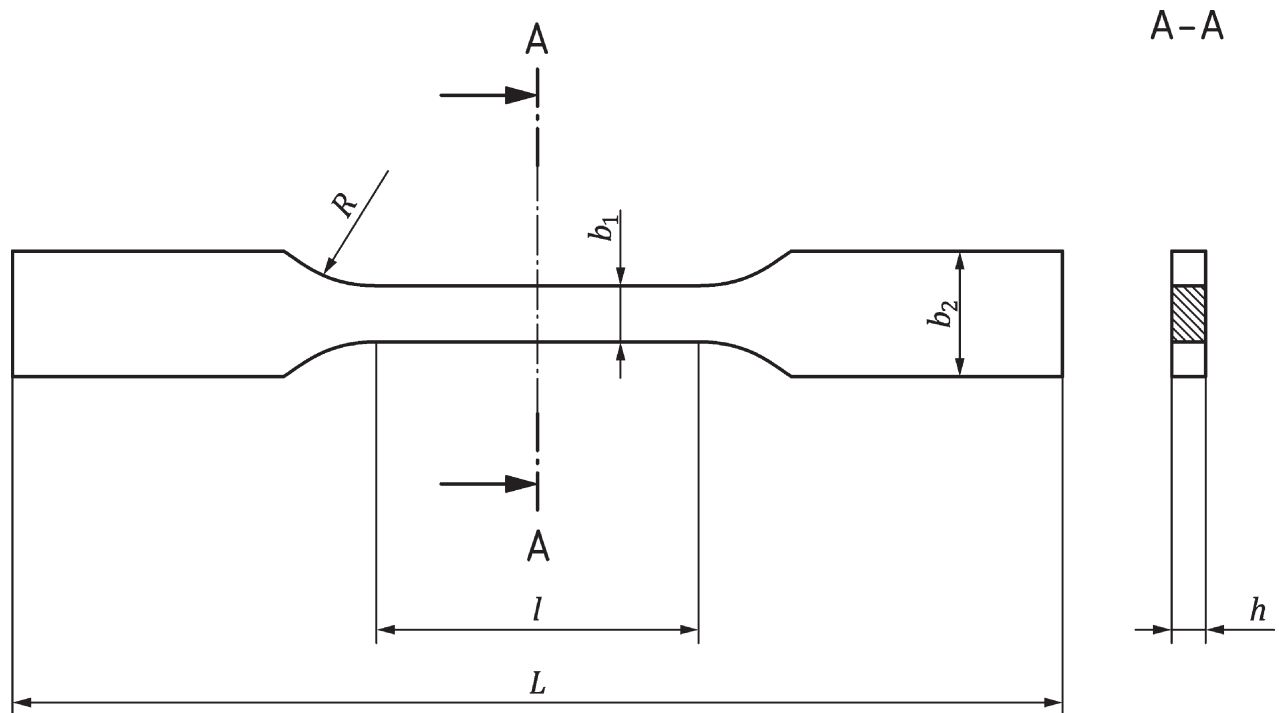
Bild 4 — Probekörper vom Typ 4
