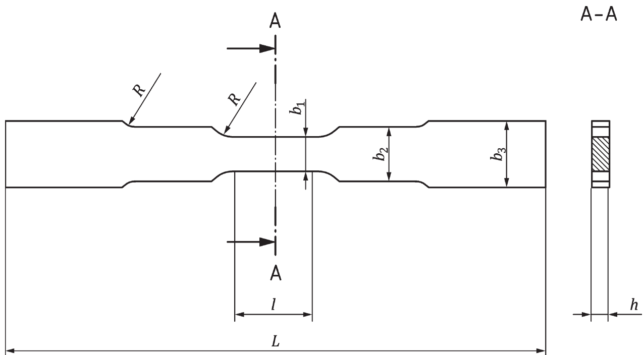
Bild 5 — Probekörper vom Typ 5
