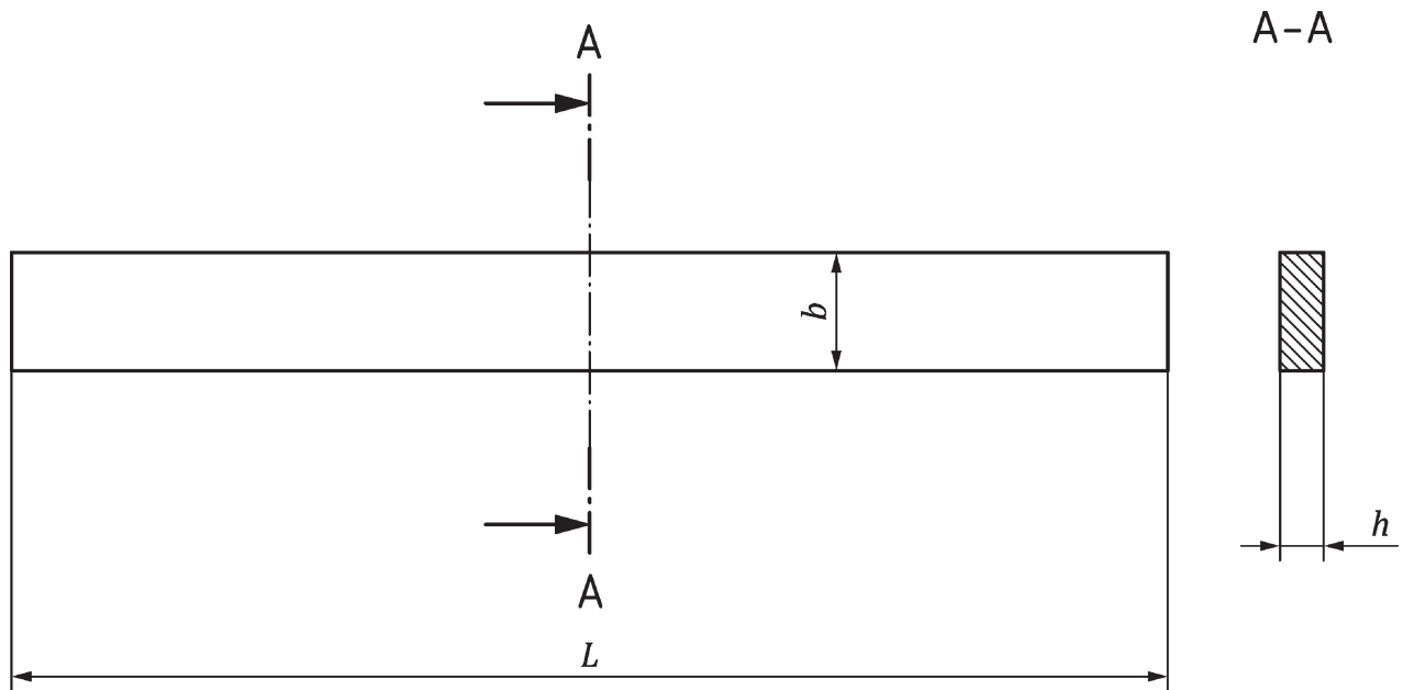
Bild 6 — Probekörper vom Typ 6
