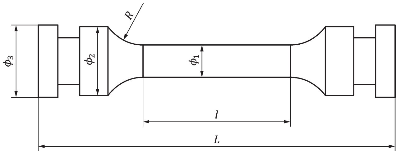
Bild 2 — Probekörper vom Typ 2
