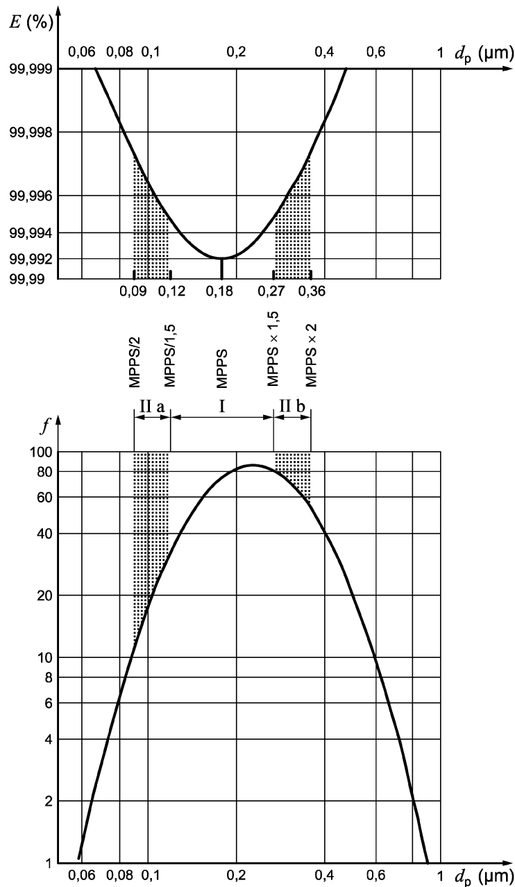
Bild 4 — Partikelgrößenbezogener Abscheidegrad, E , und zulässige Messbereiche relativ zum Abscheidegradminimum (MPPS gleich 0,18 \mu\text{m} ) und Anzahlverteilung, f , eines polydisperses Prüfaerosols mit d_p gleich 0,23 \mu\text{m}
