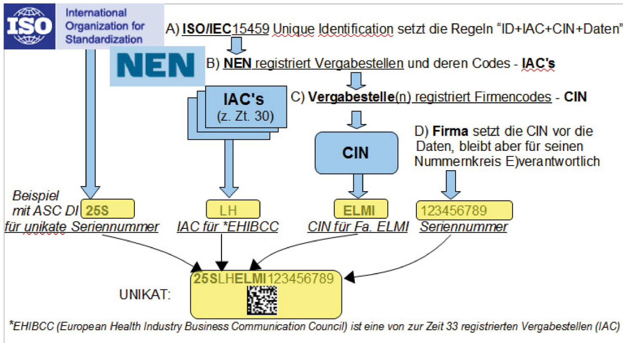
Bild 5 — Hierarchie der Eindeutigkeit und Unverwechselbarkeit für die Automatische Datenerfassung
