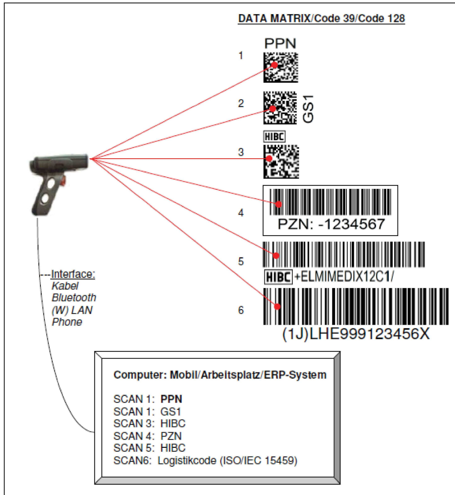
Bild 6 — Mischung von ISO ASC und GS1 Formaten (Quelle IFA-Coding-System)
