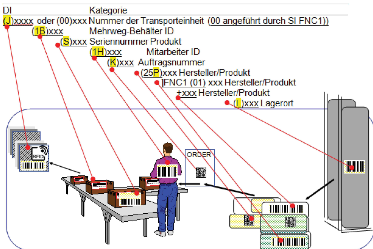
Bild 4 — Anwendung von Identifikatoren mit einer Auswahl von DIs, AIs und SIs im Verbund
