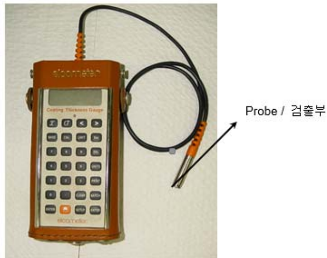
Figure 1: Dry Film Thickness Gauge / 그림 1: Dry Film Thickness Gauge
