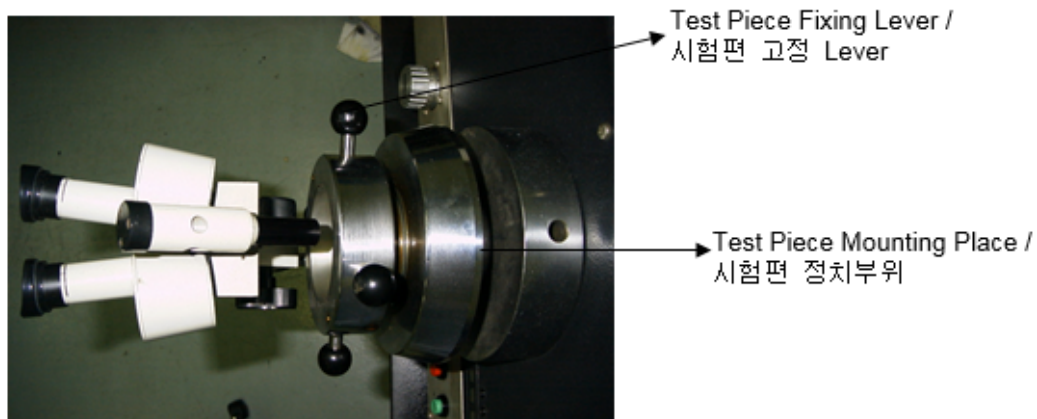
Figure 2: Cupping Tester (Side) / 그림 2: Cupping Tester (측면)
