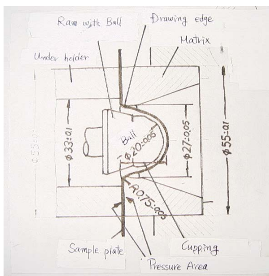
Figure 3: Steel Ball / 그림 3: Steel Ball
