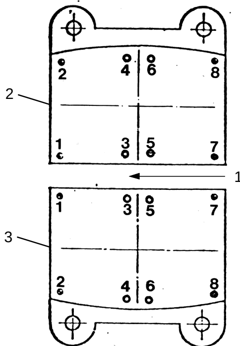
Abb. 2: Bremsbelagverschleiß - Meßpunktlage bei Scheibenbremsen
