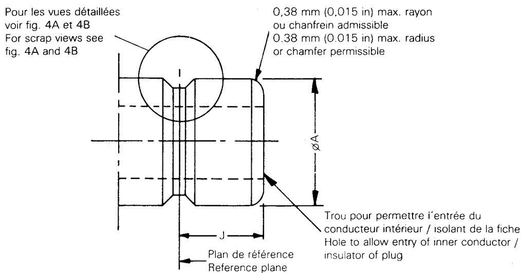
FIG. 4. — Calibres pour le contact extérieur de la fiche. Gauges for outer contact of plug.
