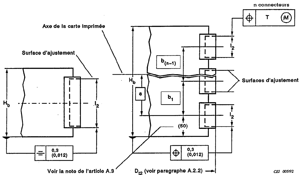
Figure 12 - Position des connecteurs sur des blocs enfichables des bacs plus grands que 3U
